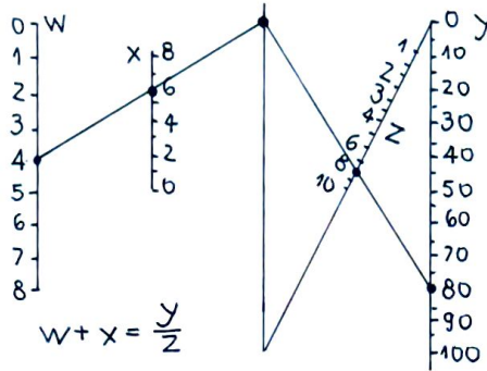
Nomograma con 4 variables
