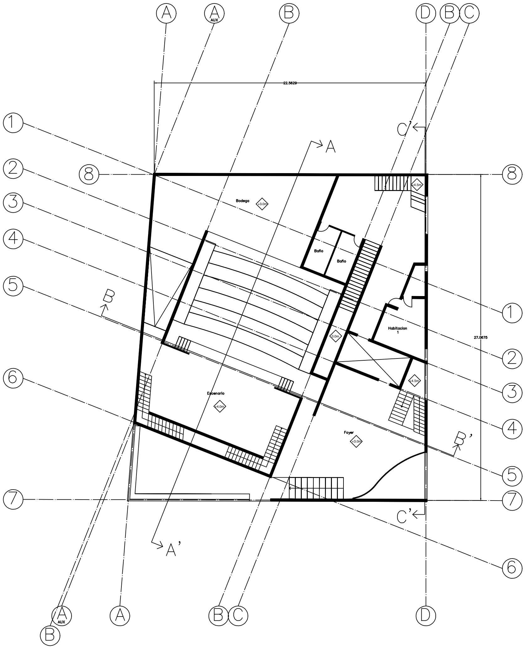
Planta 1
