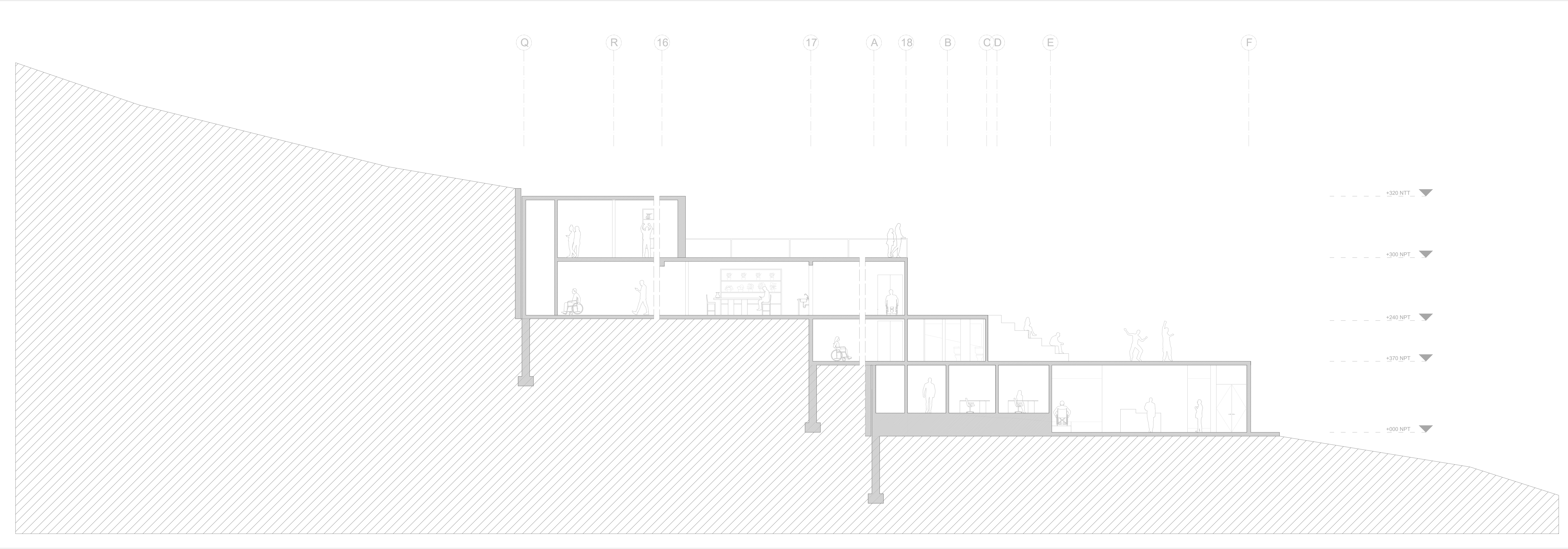
Corte B -B' Escala 1 / 100
