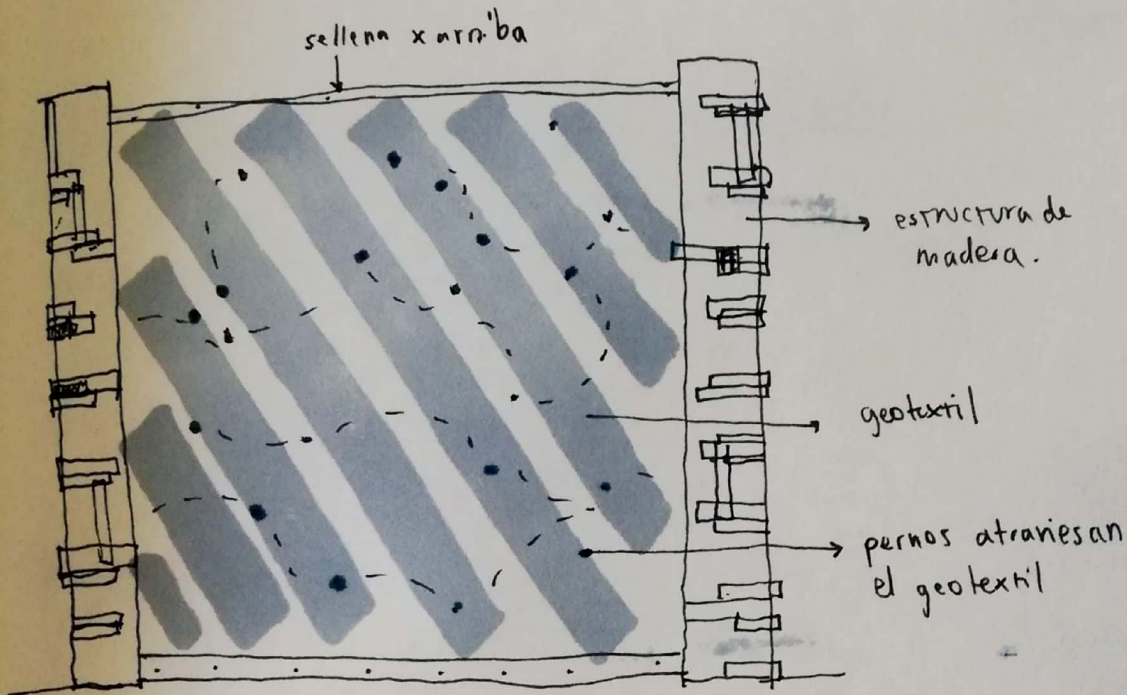
ELEVACION ESQUEMÁTICA.
