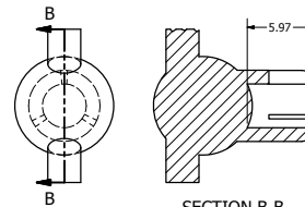
SECTION B-B SCALE 4 : 1
