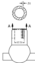
SECTION A-A SCALE 4 : 1
