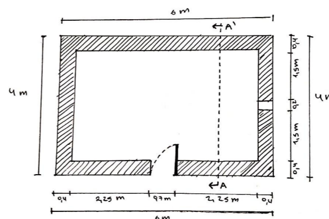
ELEVACION ESC: 1:50 VIVIENDA HUILLOC
