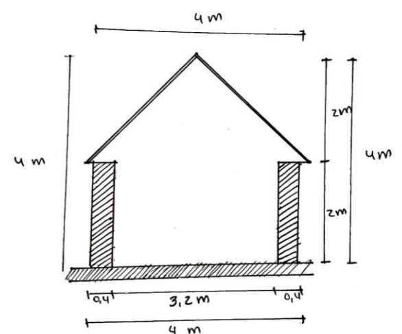
CORTE A-A' ESC: 1:50 VIVIENDA HUILLOC
