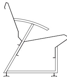
1995 Banca de metal Juan Carlos Jeldes Banca de una plancha de acero {Ficha p.43}
