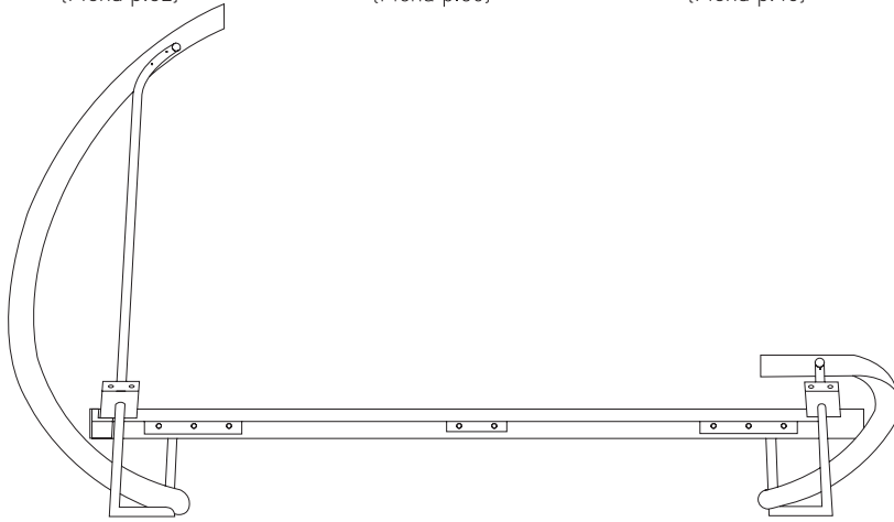
1982 Silla para la capilla de Ritoque Raul Celis Asiento de ferro-cemento y asbesto-cemento con uniones de madera {Ficha p.28}
