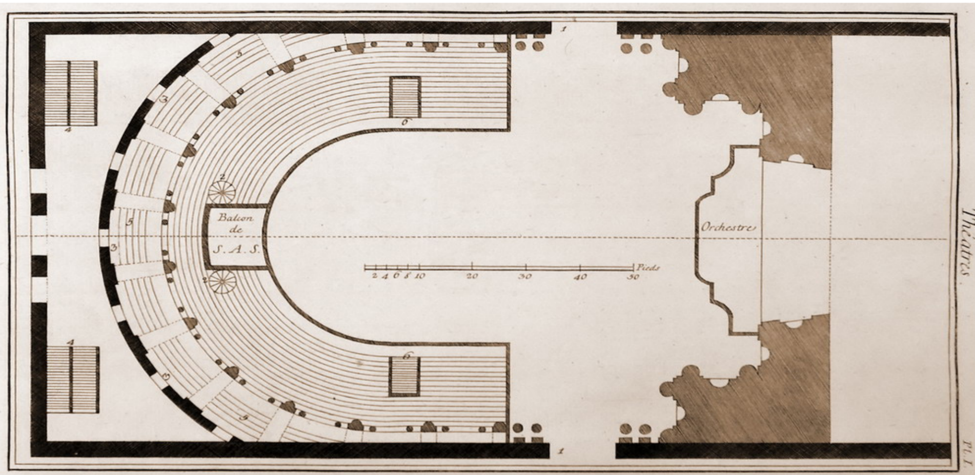
Planta del teatro
