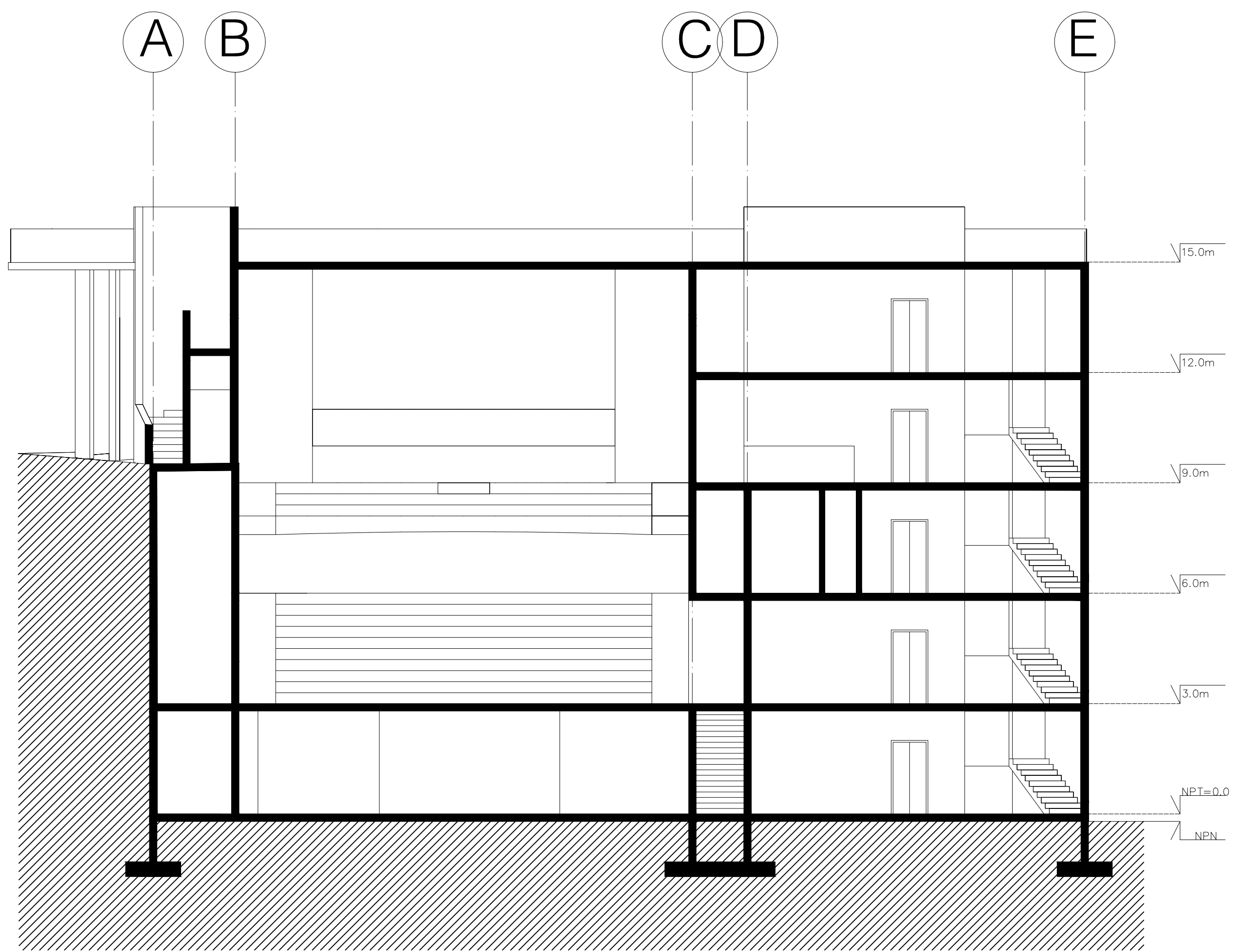
corte B-B'
