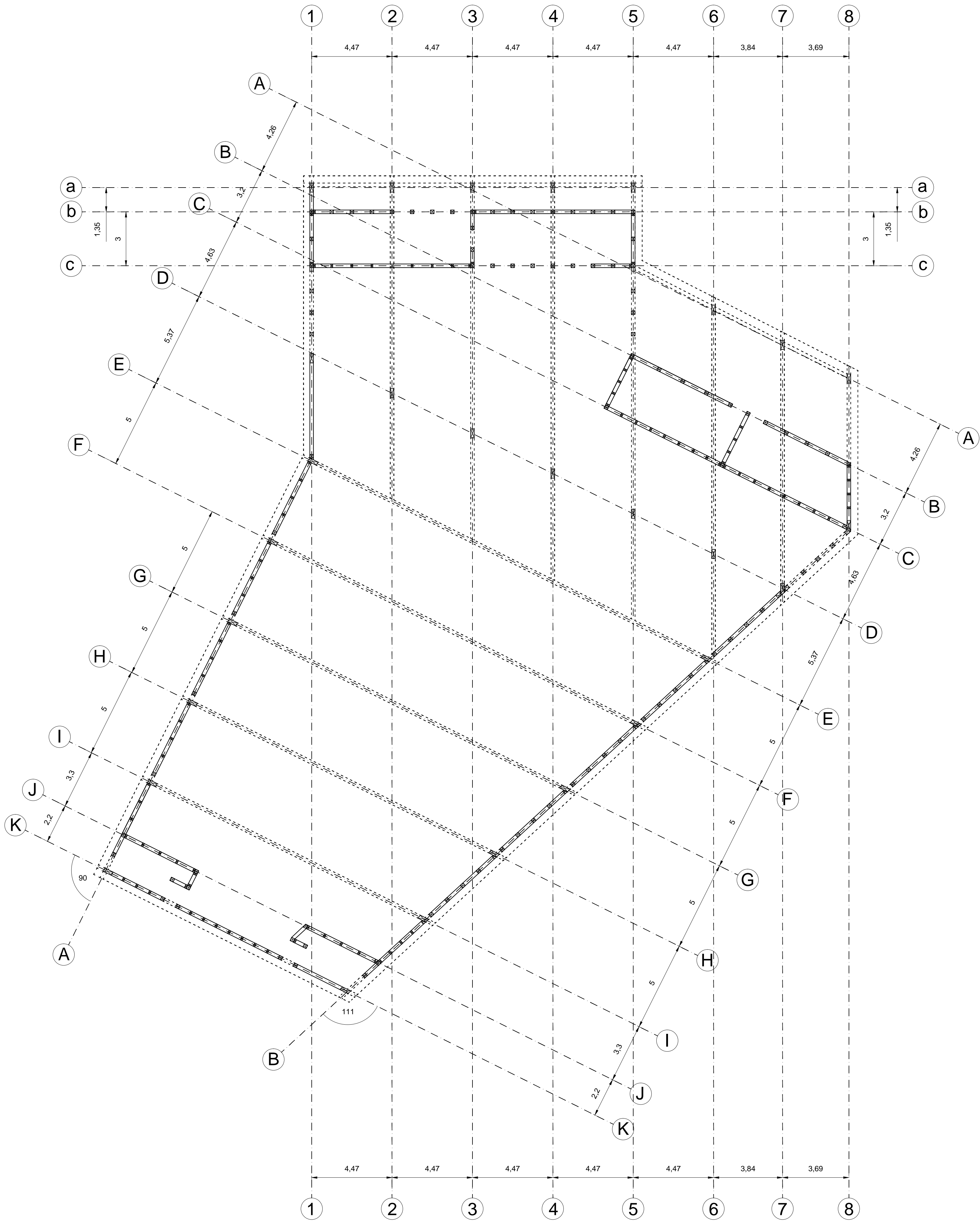
PLANTA ESTRUCTURAL ESCALA 1:125
