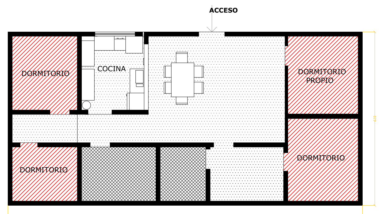
PLANTA DE RELACIÓN DORMITORIOS-VIVIENDA
