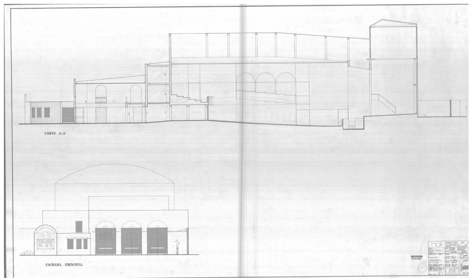
Plano Elevacion
