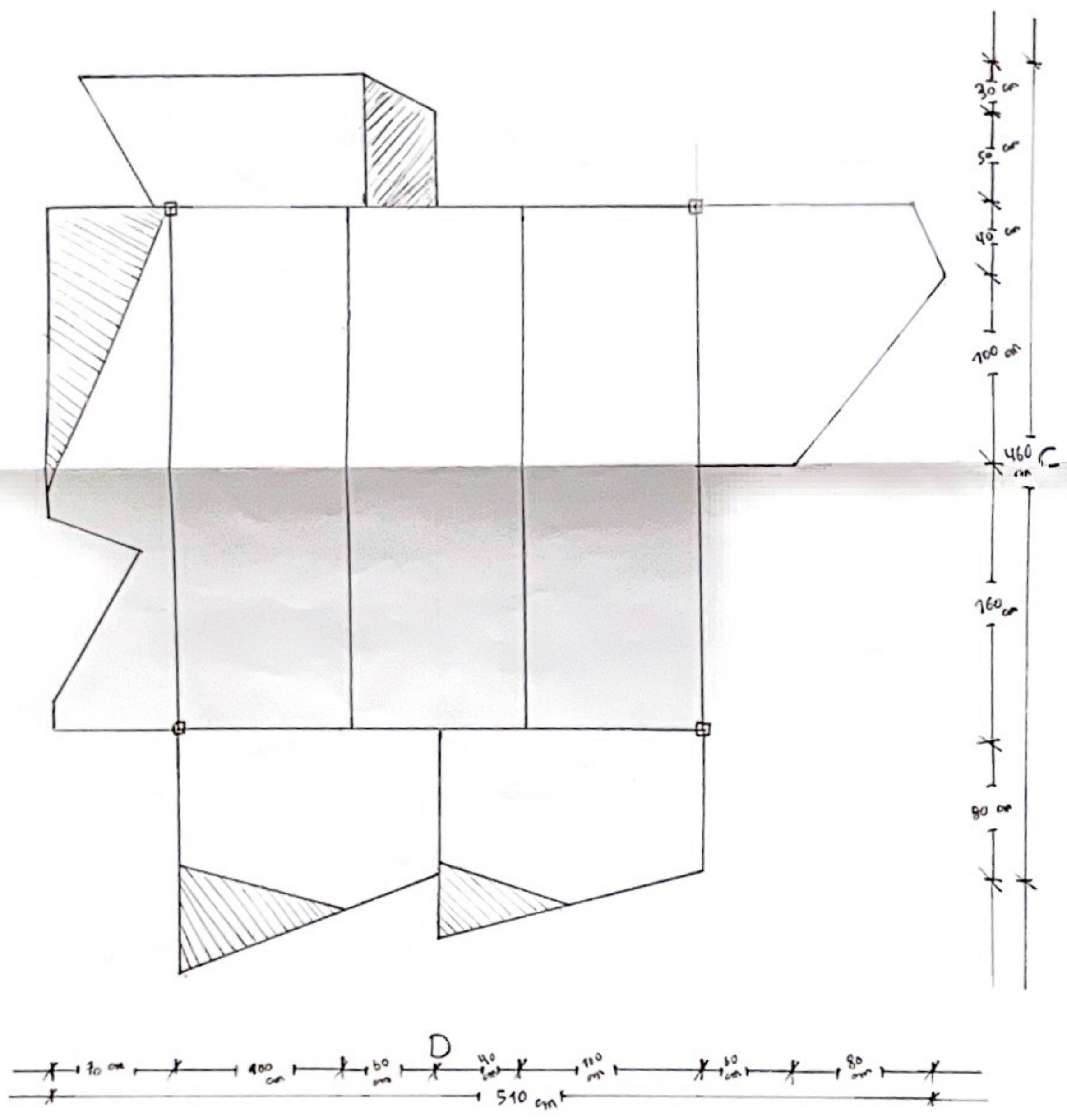
Elevación D ESC 1:20
