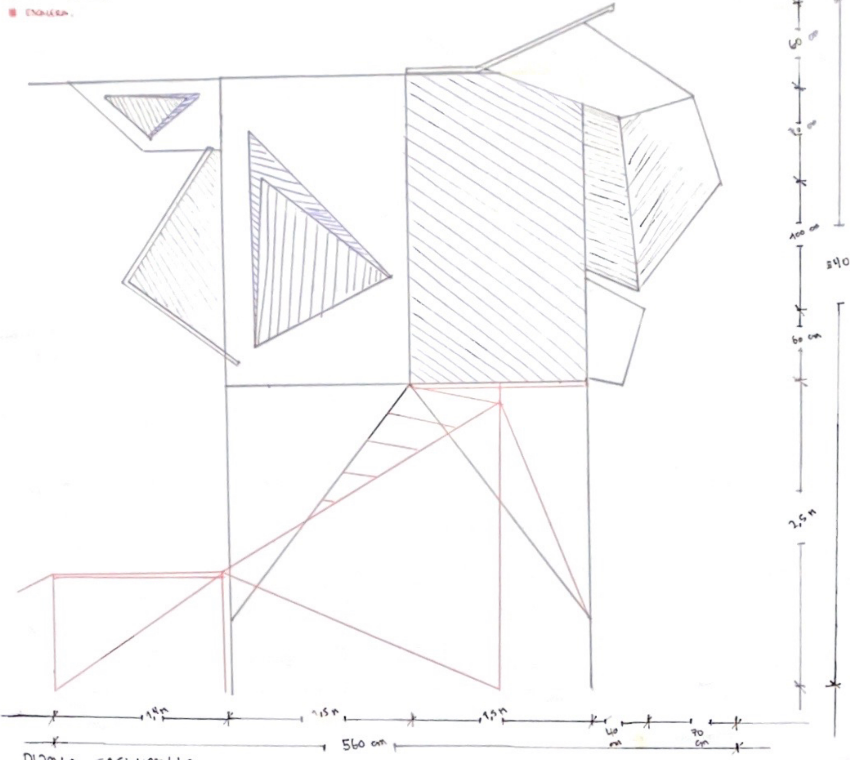
Planta techumbre ESC 1:20
