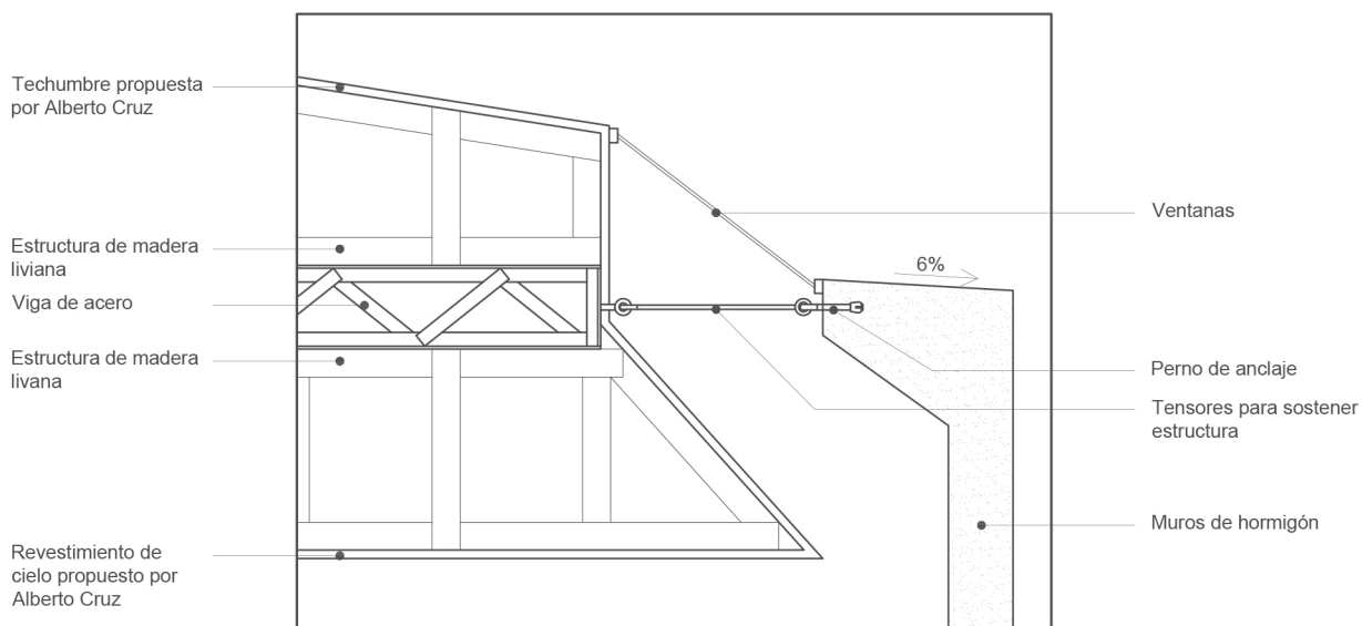
Desarrollo detalles propuesta grupal estructura de las ventanas
