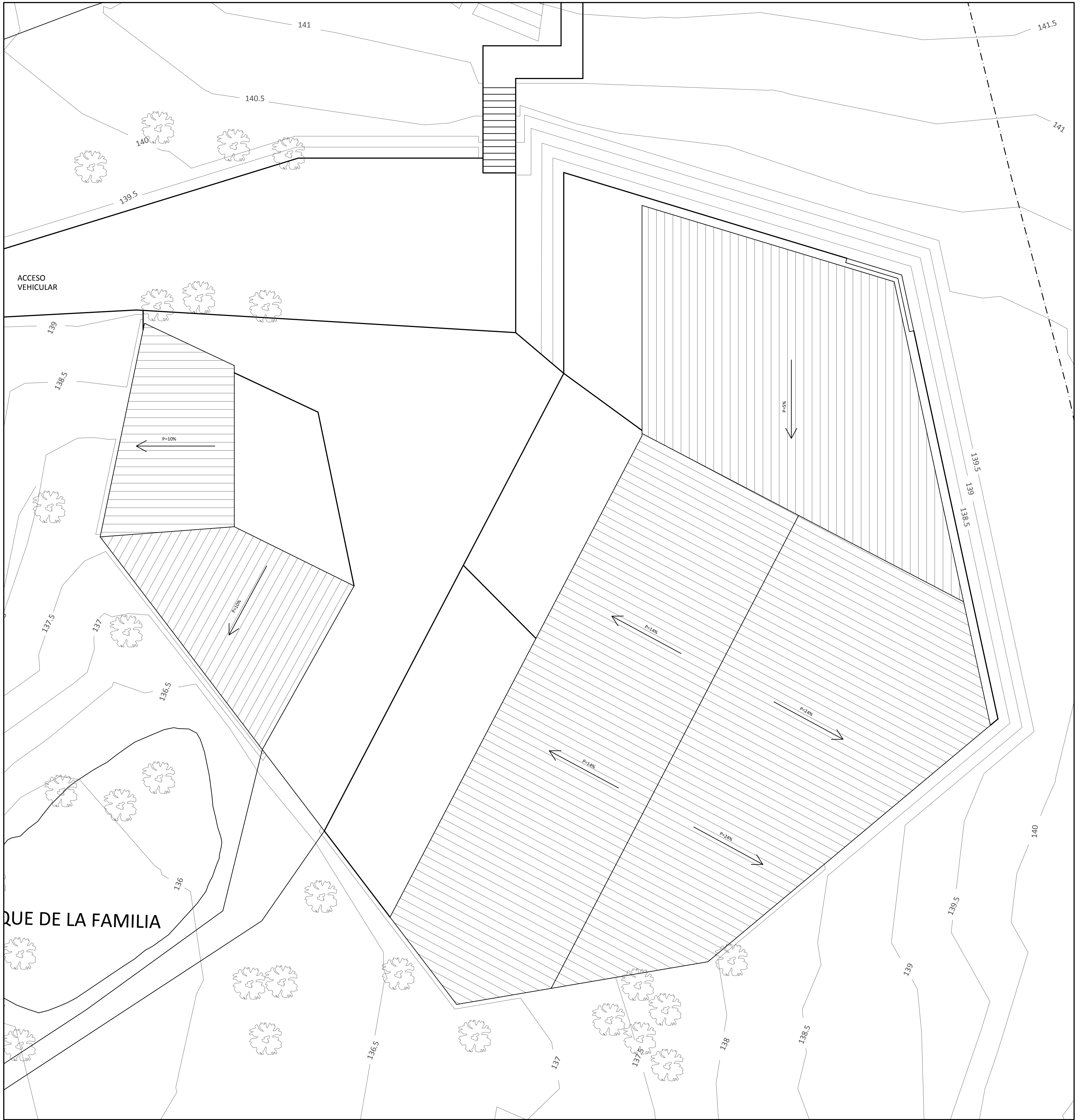
PLANO DE CUBIERTAS
