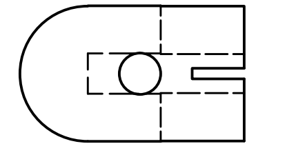
Pieza pivote superior ESCALA 2 : 1
