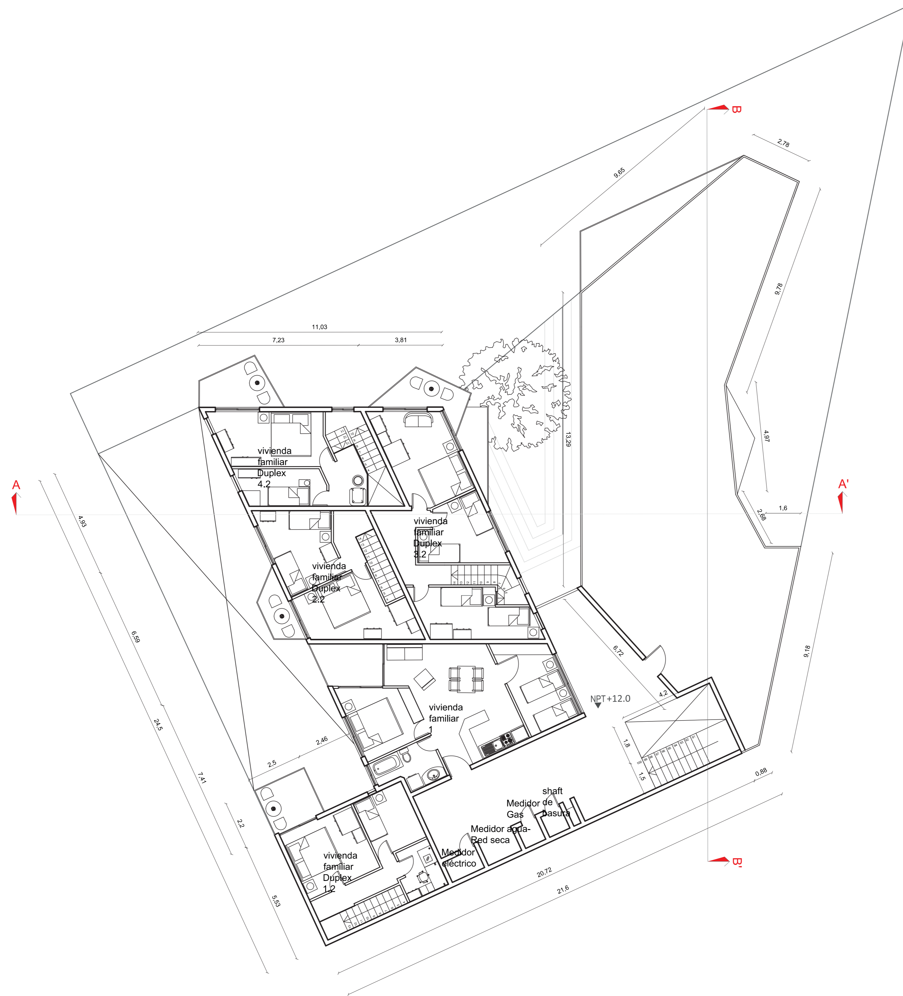
PLANTA N° 5 ESCALA 1: 100
