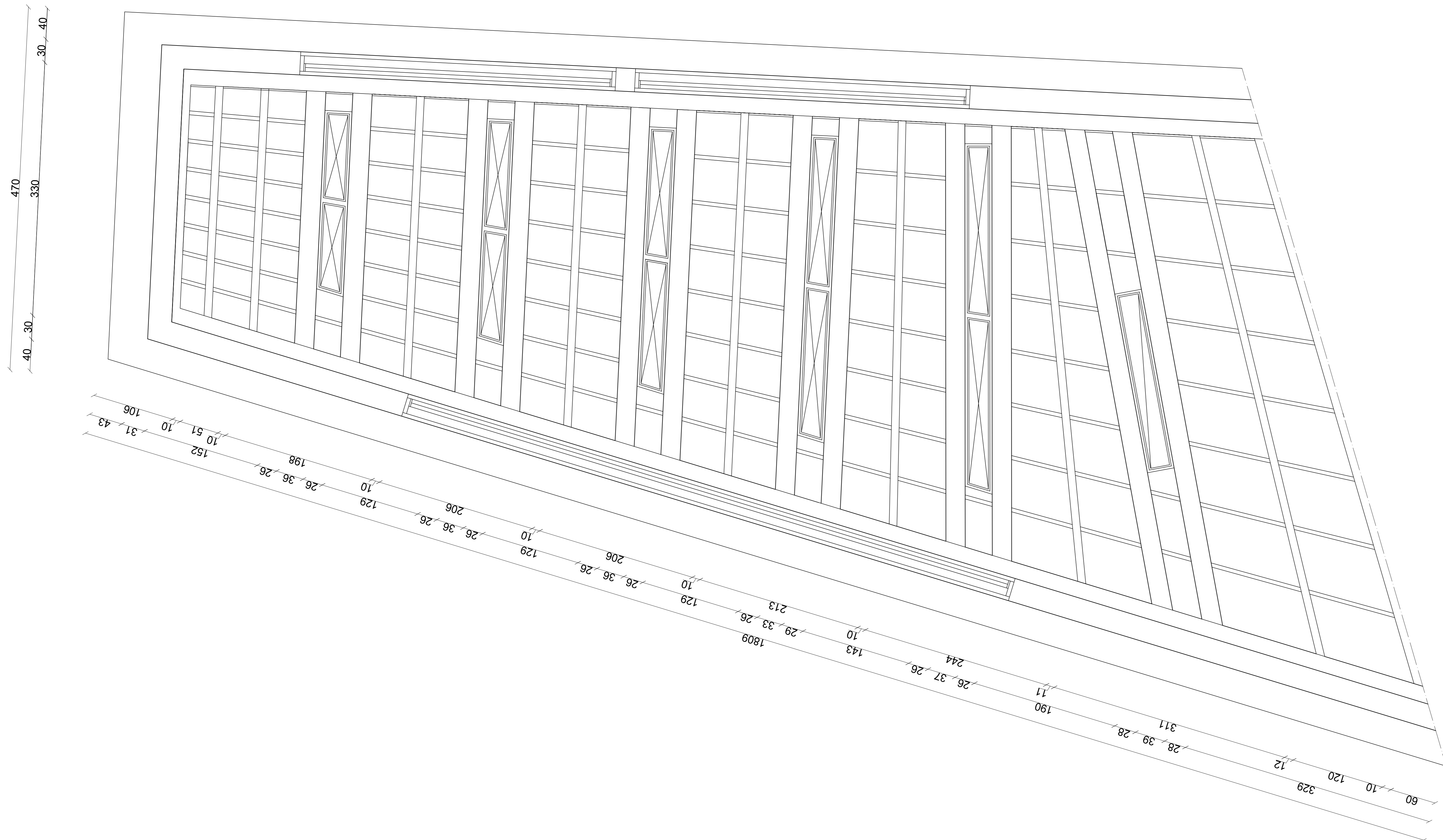
PLANTA CUBIERTA INTERIOR ESCALA. 1/20
