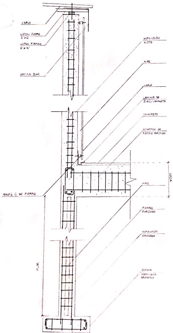
Escantillón 1:10
