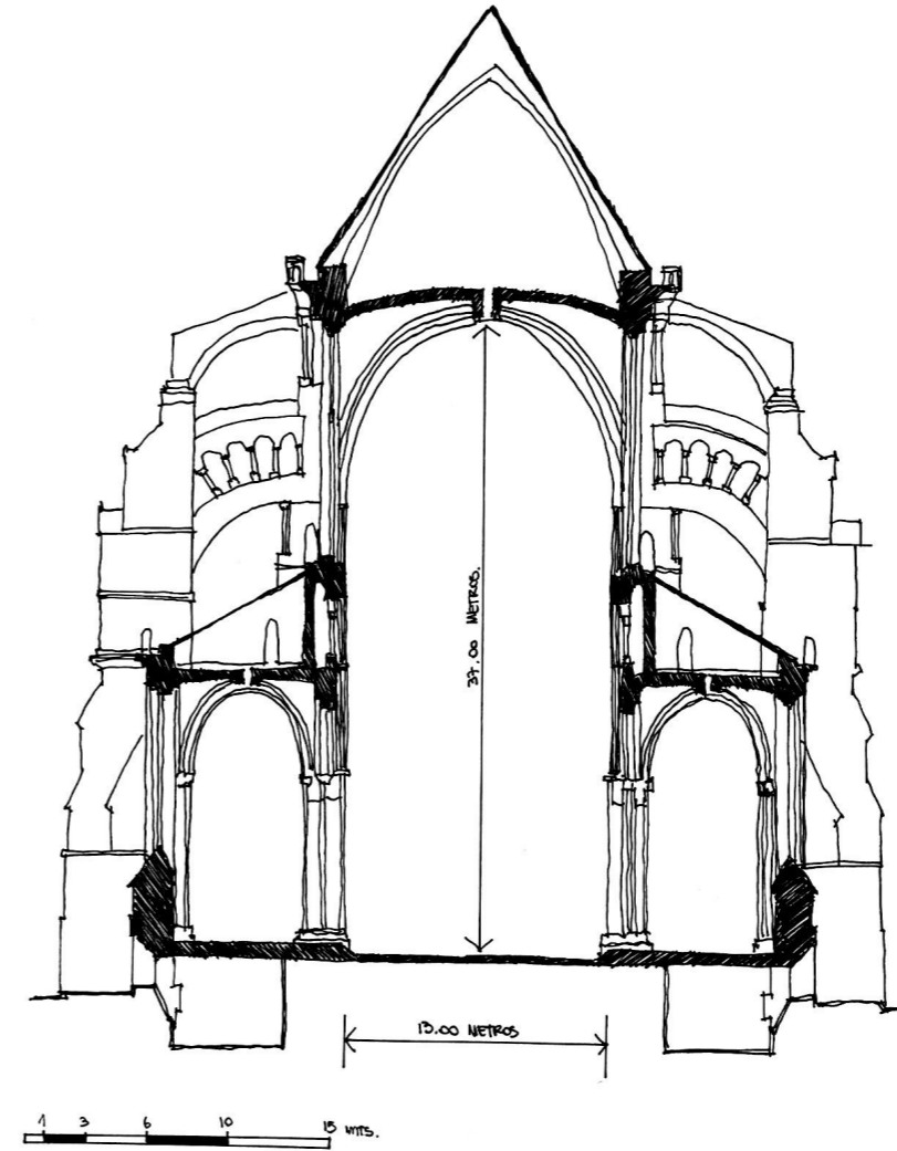
2/ Corte Transversal
