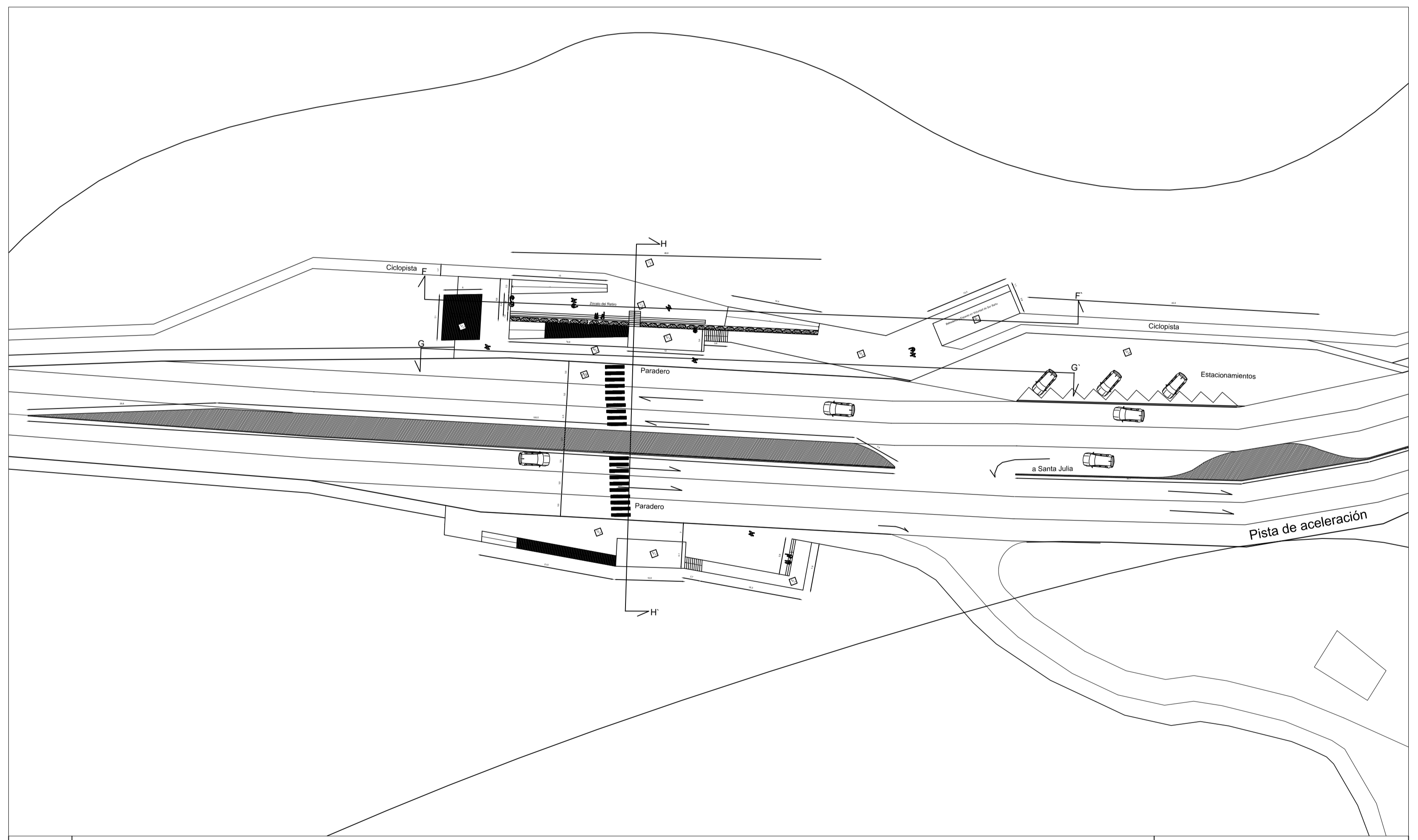
RUTA F30E, SECTOR SANTA JULIA PLANTA DE CRUCE-ACCESO A SANTA JULIA / PROPUESTA DE PARADERO PASEO MIRADOR ESCALA 1:500
