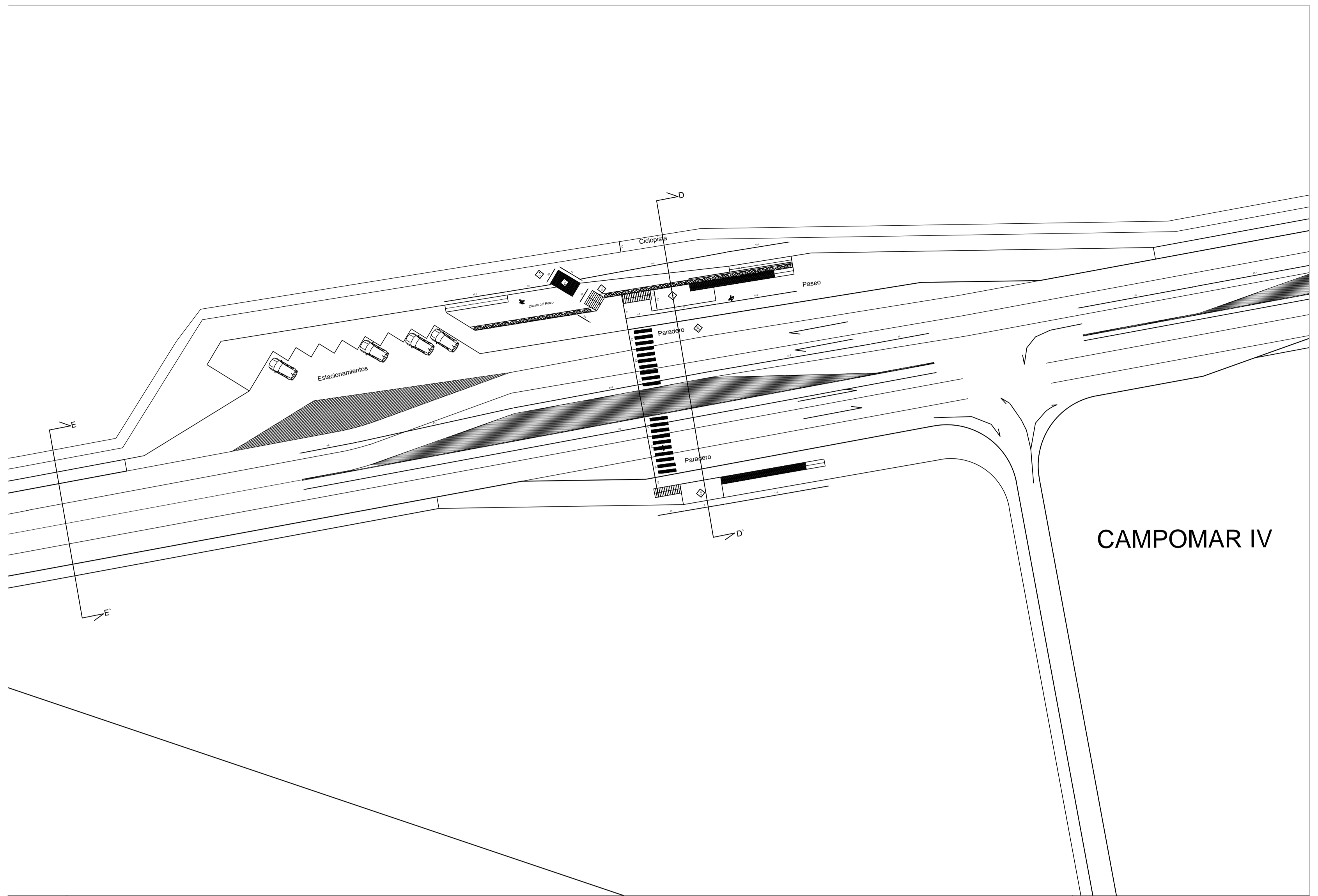
RUTA F30E, SECTOR ACCESO A CONDOMINIO CAMPOMAR IV PLANTA DE CRUCE CAMPOMAR IV / PROPUESTA DE PARADERO PASEO MIRADOR ESCALA 1:500
