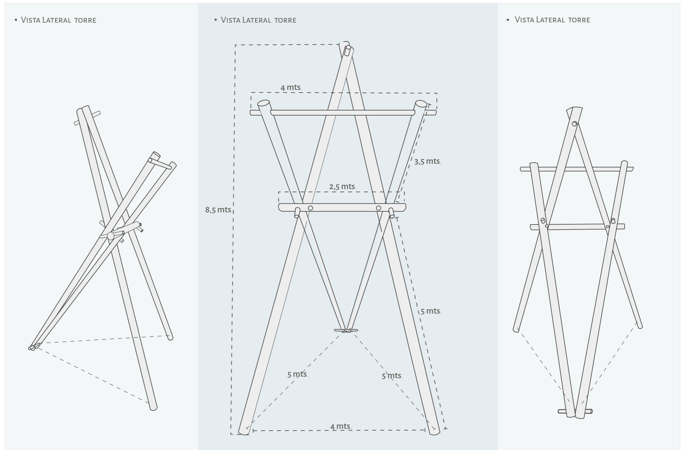
° Dibujos lineales de la maqueta a escala de la torre . ( Las medidas expuestas en el dibujo, son las medidas reales de la estructura).
