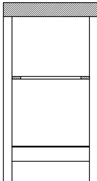
B-B ( 1 : 10 )
