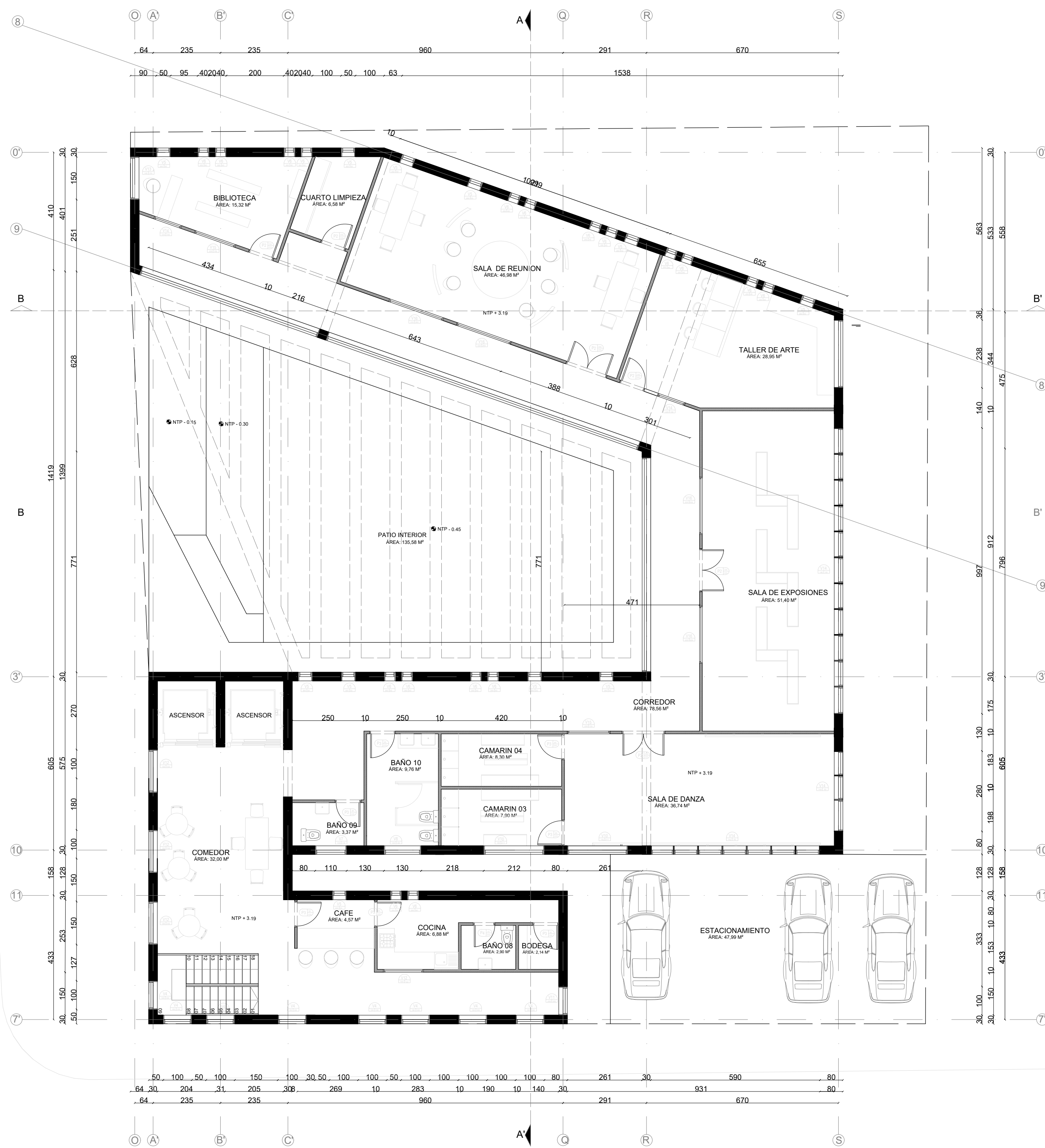
PLANTA ARQUITECTÓNICA NIVEL +3,19 Escala 1:100
