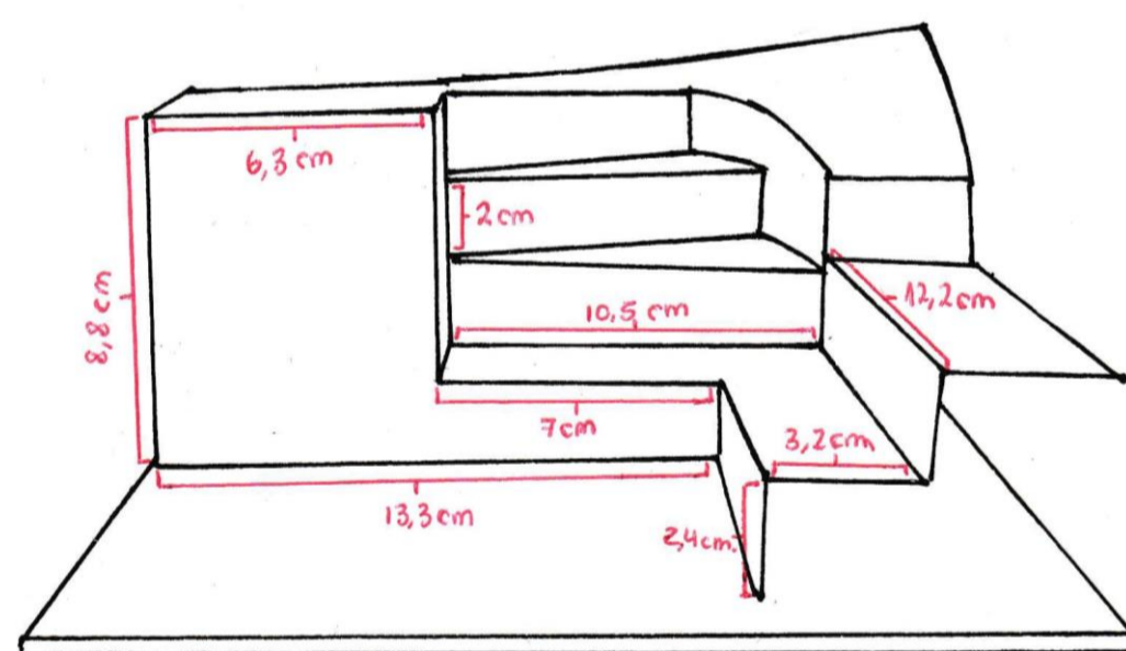
*Esquema Maqueta
