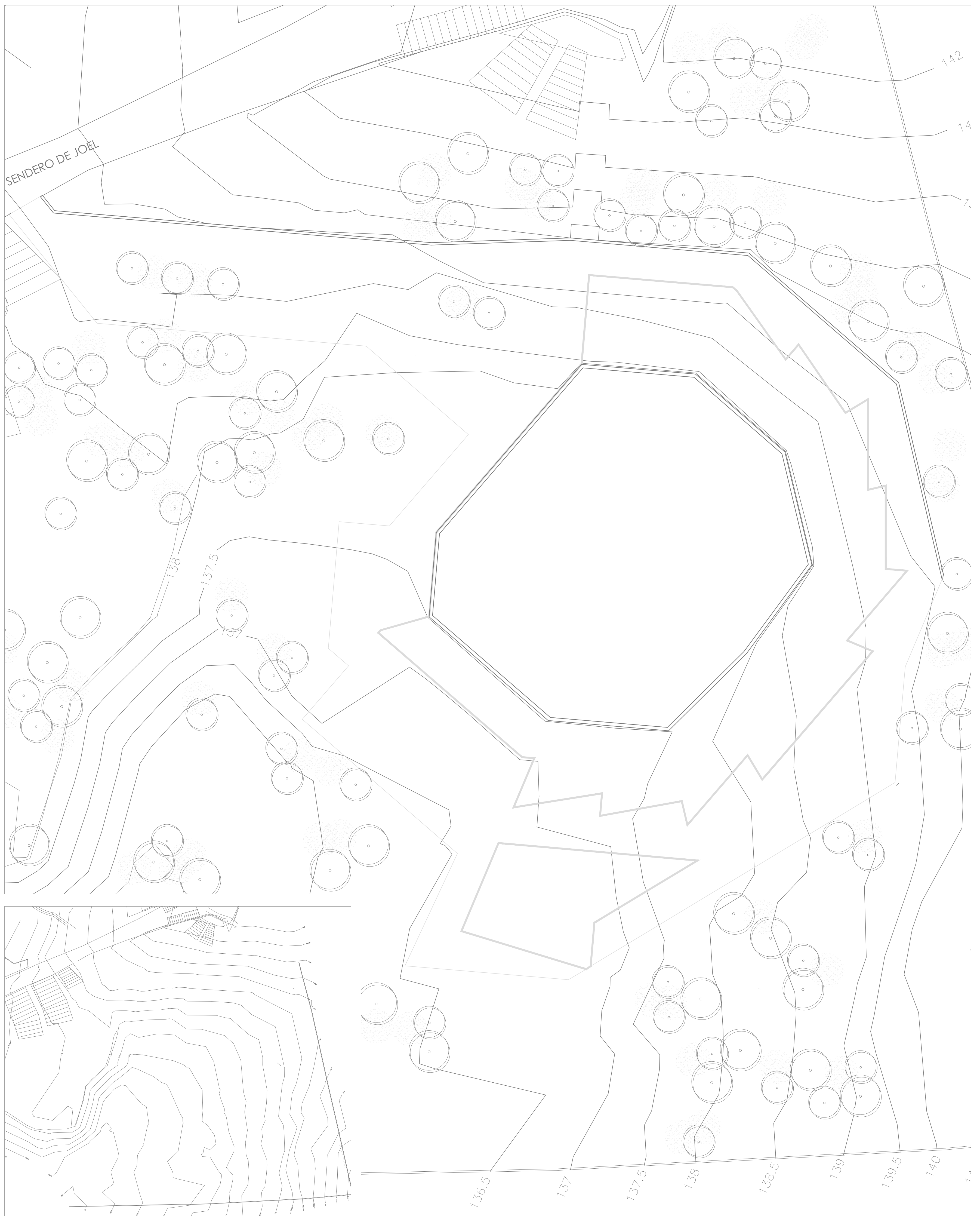
SITUACION ACTUAL TERRENO NATURAL Esc.: 1:500
