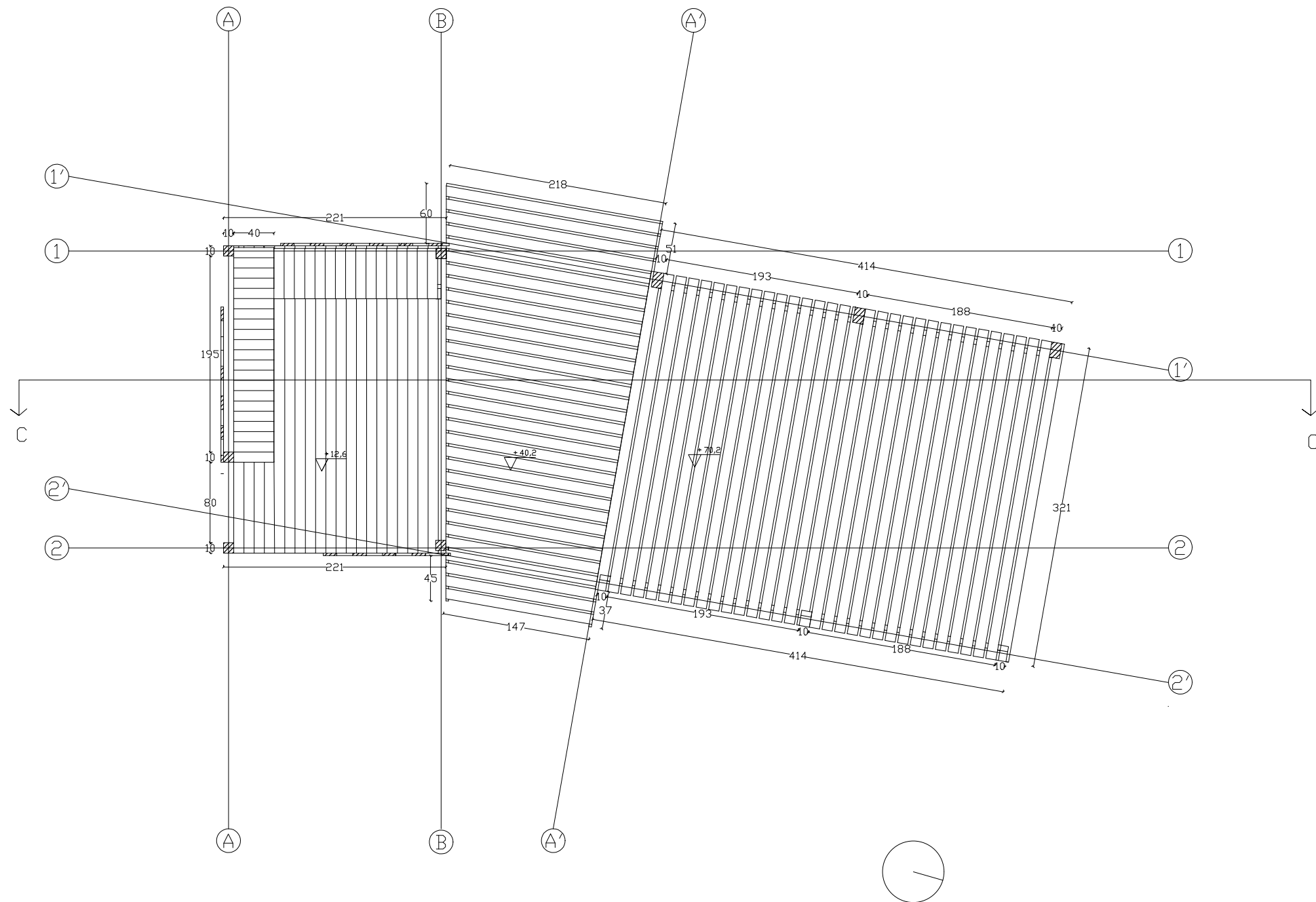
PLANTA 1:200
