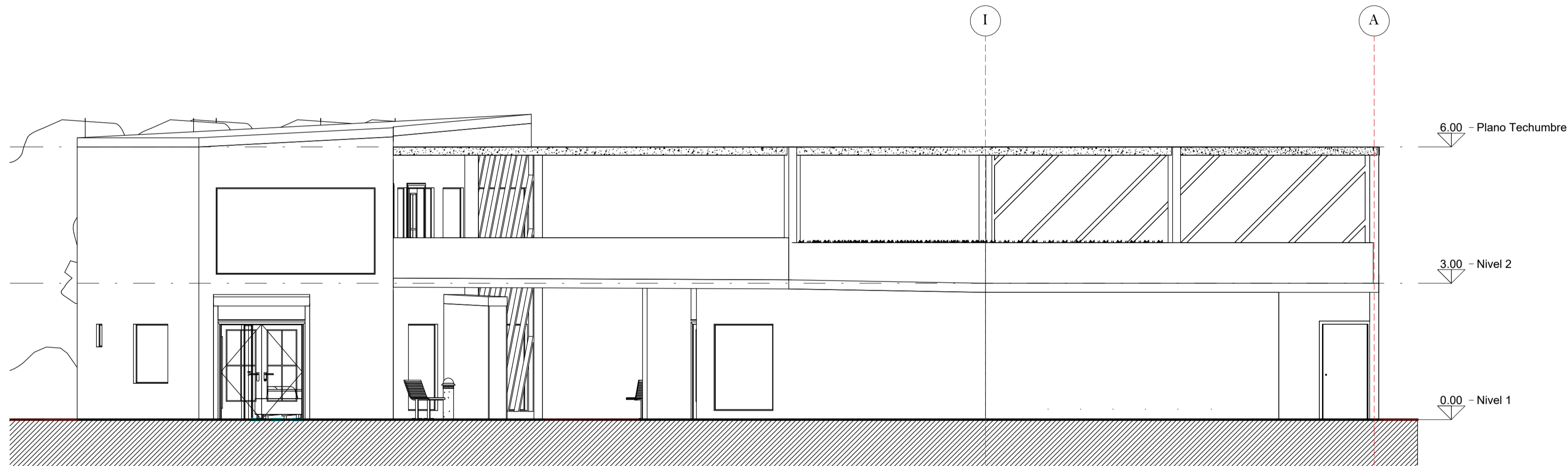
Elevación Sur 1 : 75
