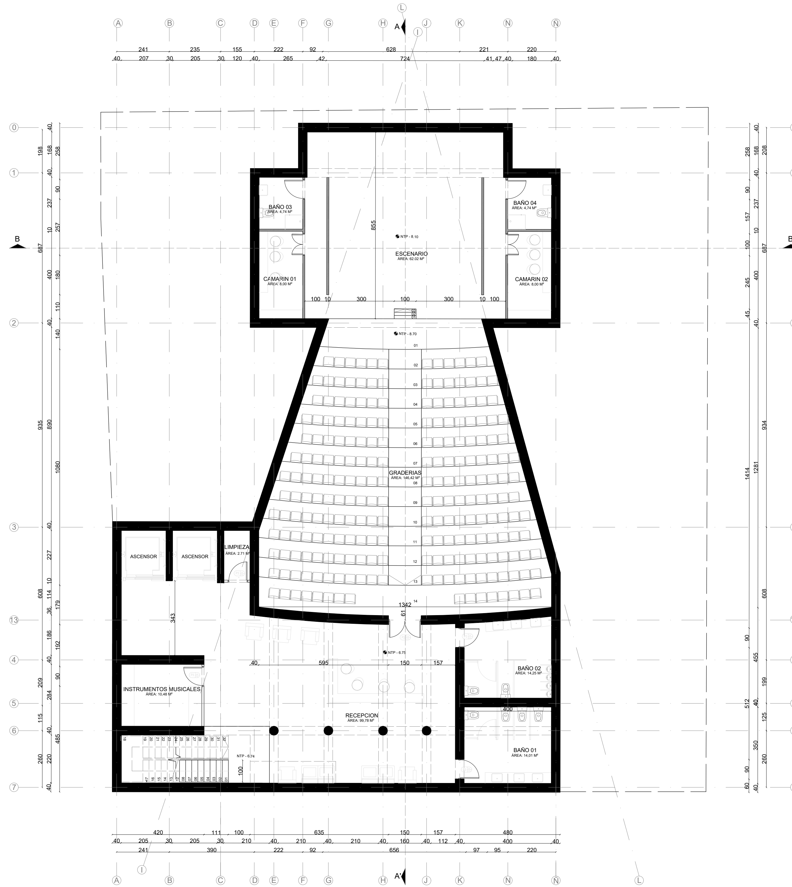
PLANTA ARQUITECTÓNICA NIVEL -6,90 Escala 1:100
