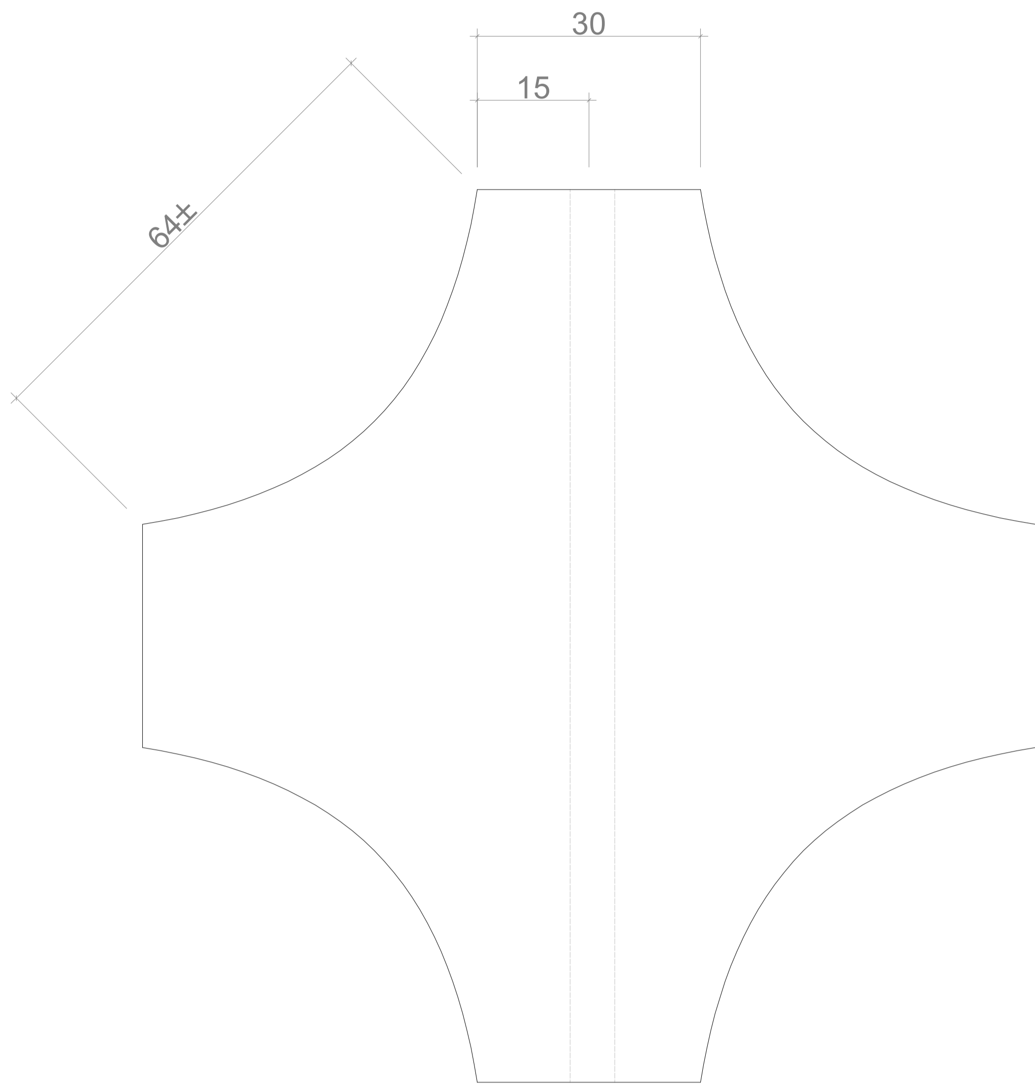
VISTA FRONTAL 2 : 1
