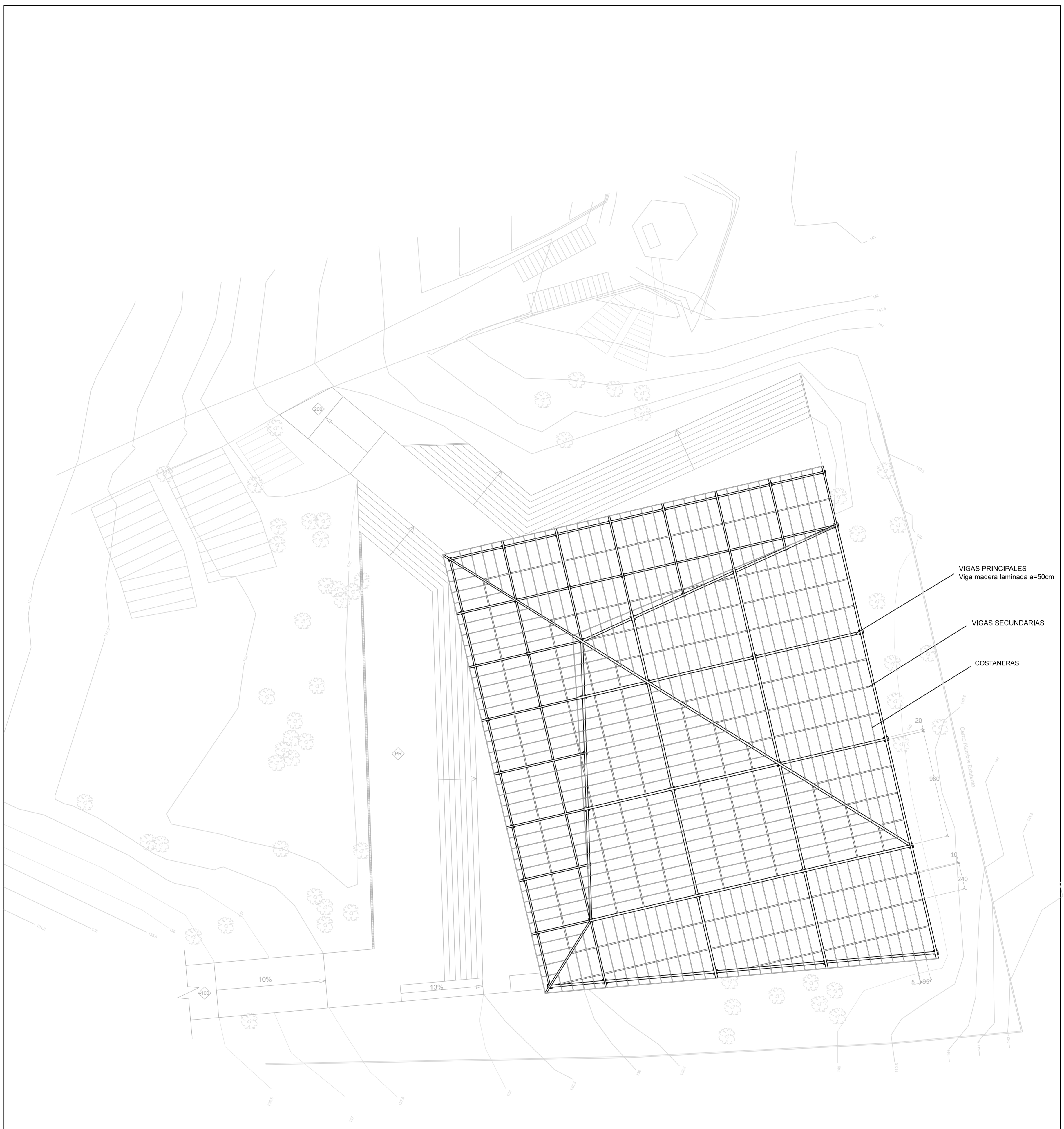
PLANTA ESTRUCTURA TECHUMBRE
