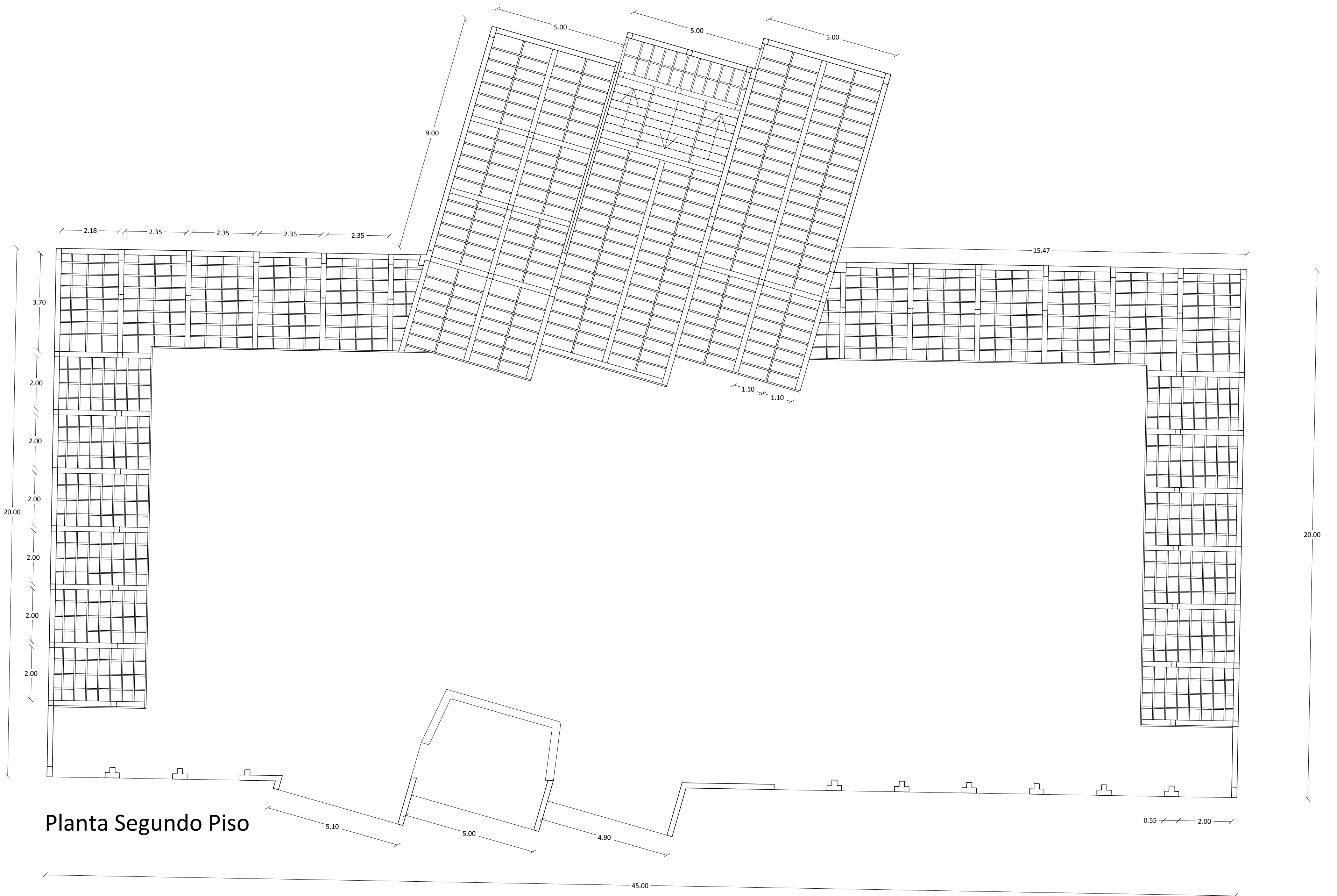
Planta Techumbre
