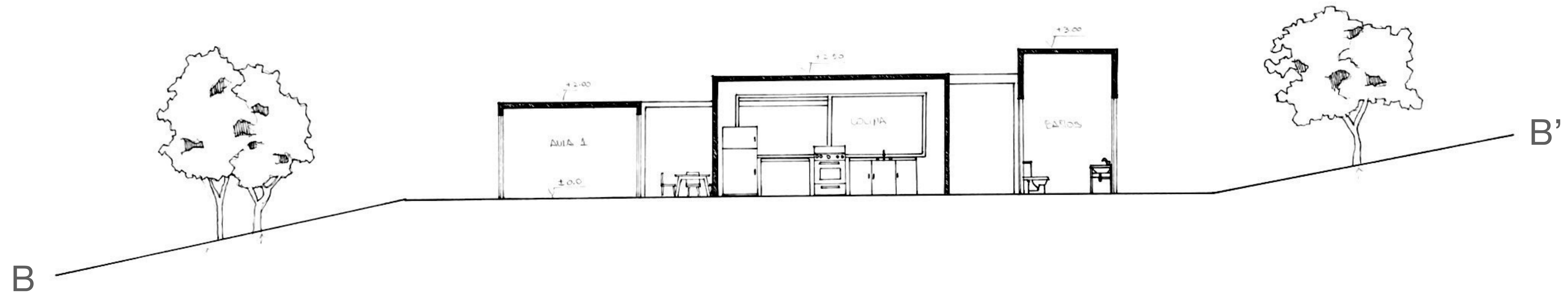
B CORTE B-B' ESCALA 1:50 COTAS EN MTS.
