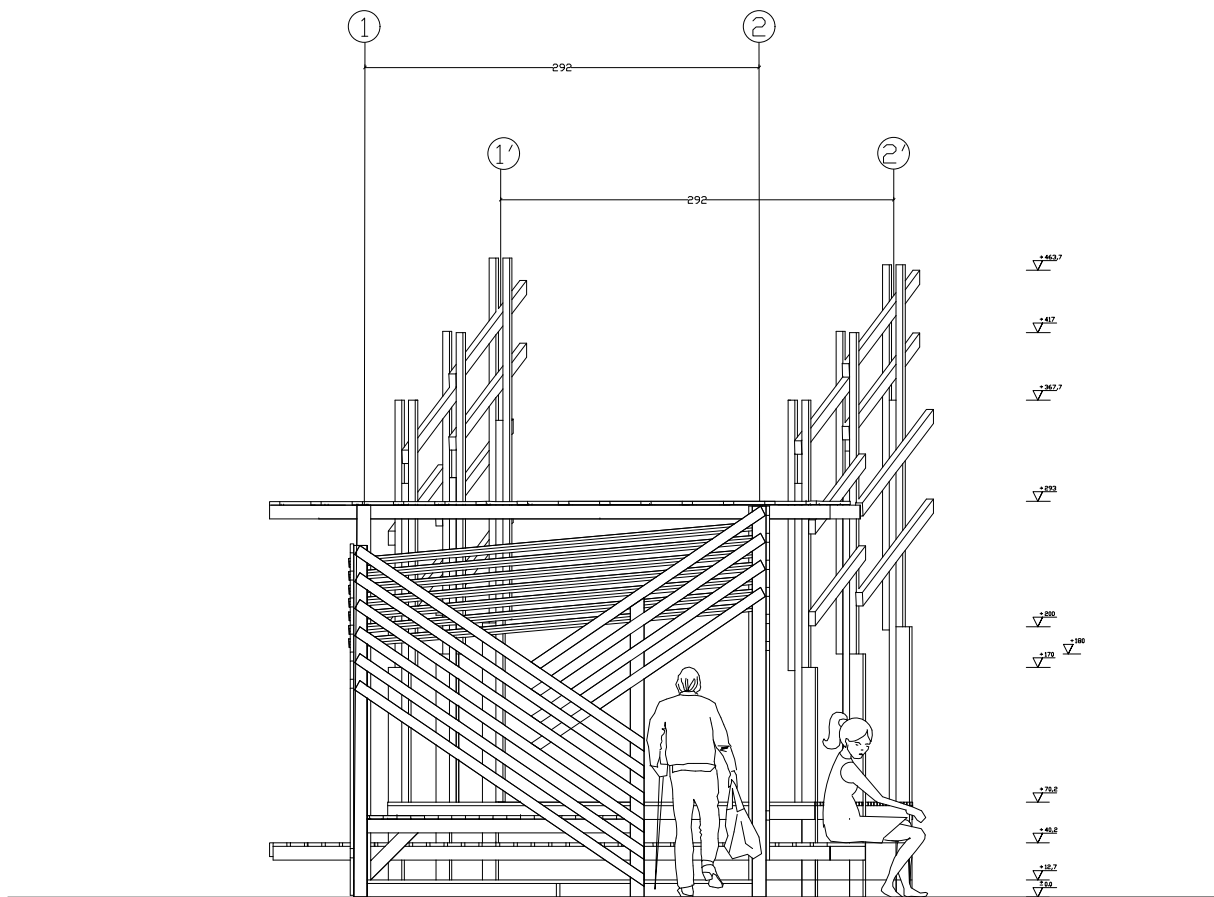
ELEVACIÓN SUR
