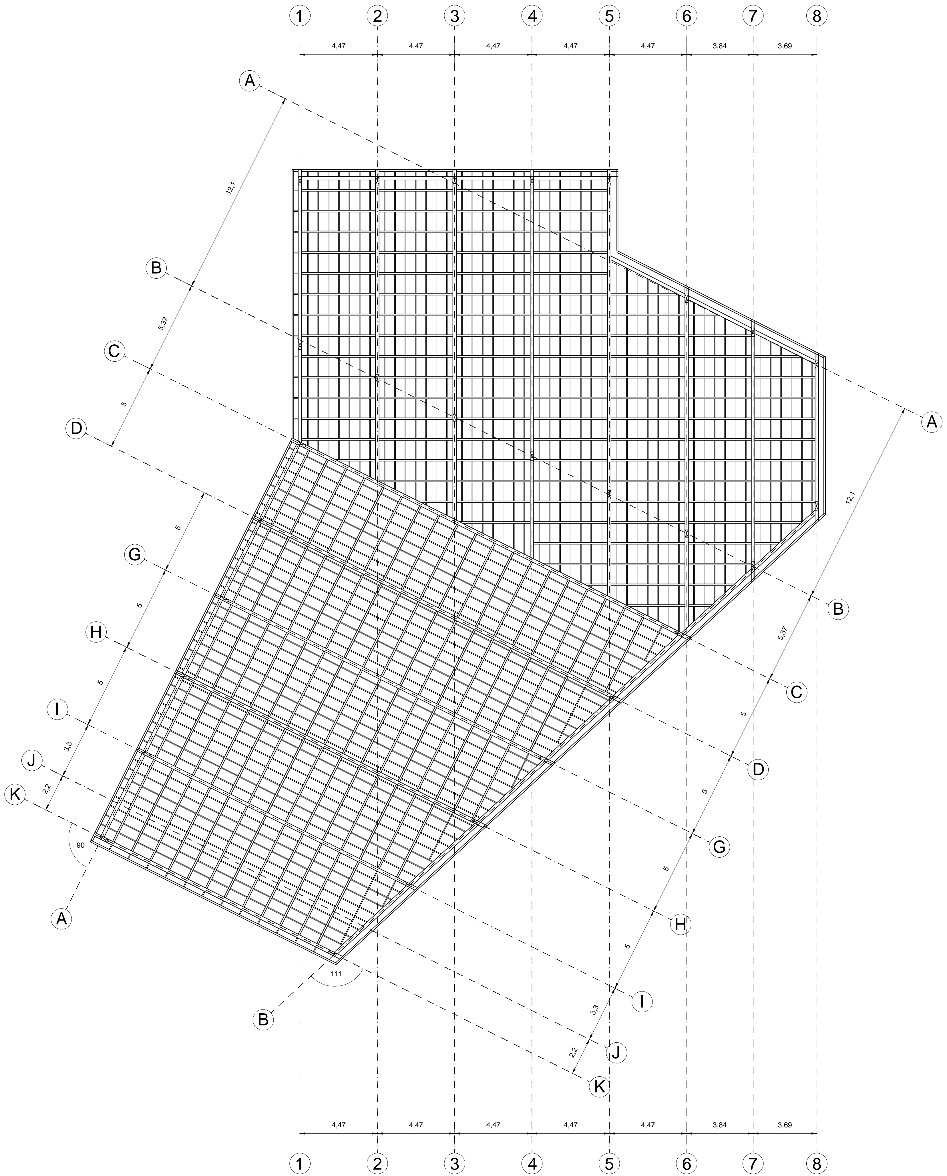
ESTRUCTURA CUBIERTA ESCALA 1:125
