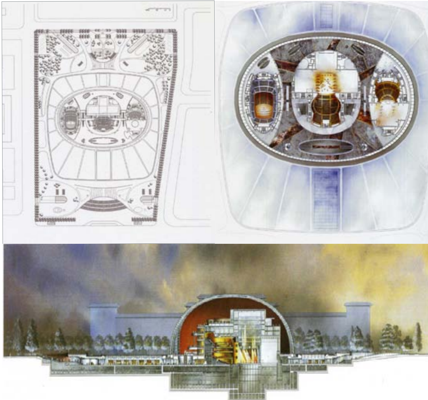
Planta arquitectónica y corte
