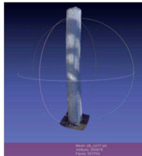
Figura 4. Levantamiento dimensional de columnas. Fuente: Centro de Patrimonio Cultural, PUC.
