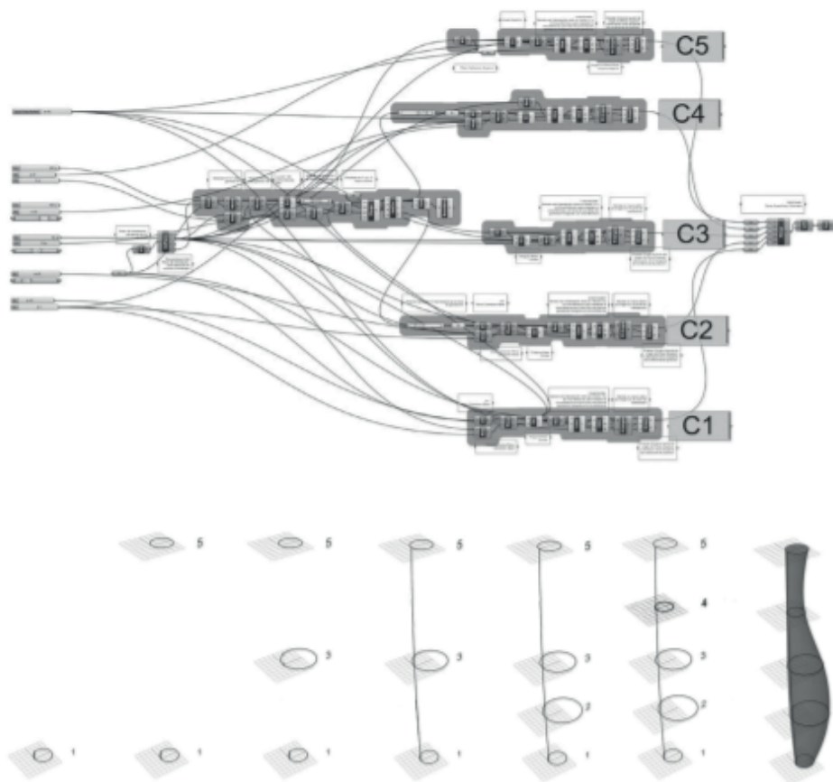
Figura 2. Programación paramétrica en Grasshopper (arriba) y estrategia de definición geométrica por circunferencias en un eje vertical (abajo). Fuente: Elaboración propia.
