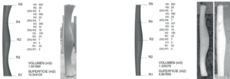
Figura 5. Comparación de modelos generados con la programación y columnas ejecutadas. Fuente: Elaboración propia.
