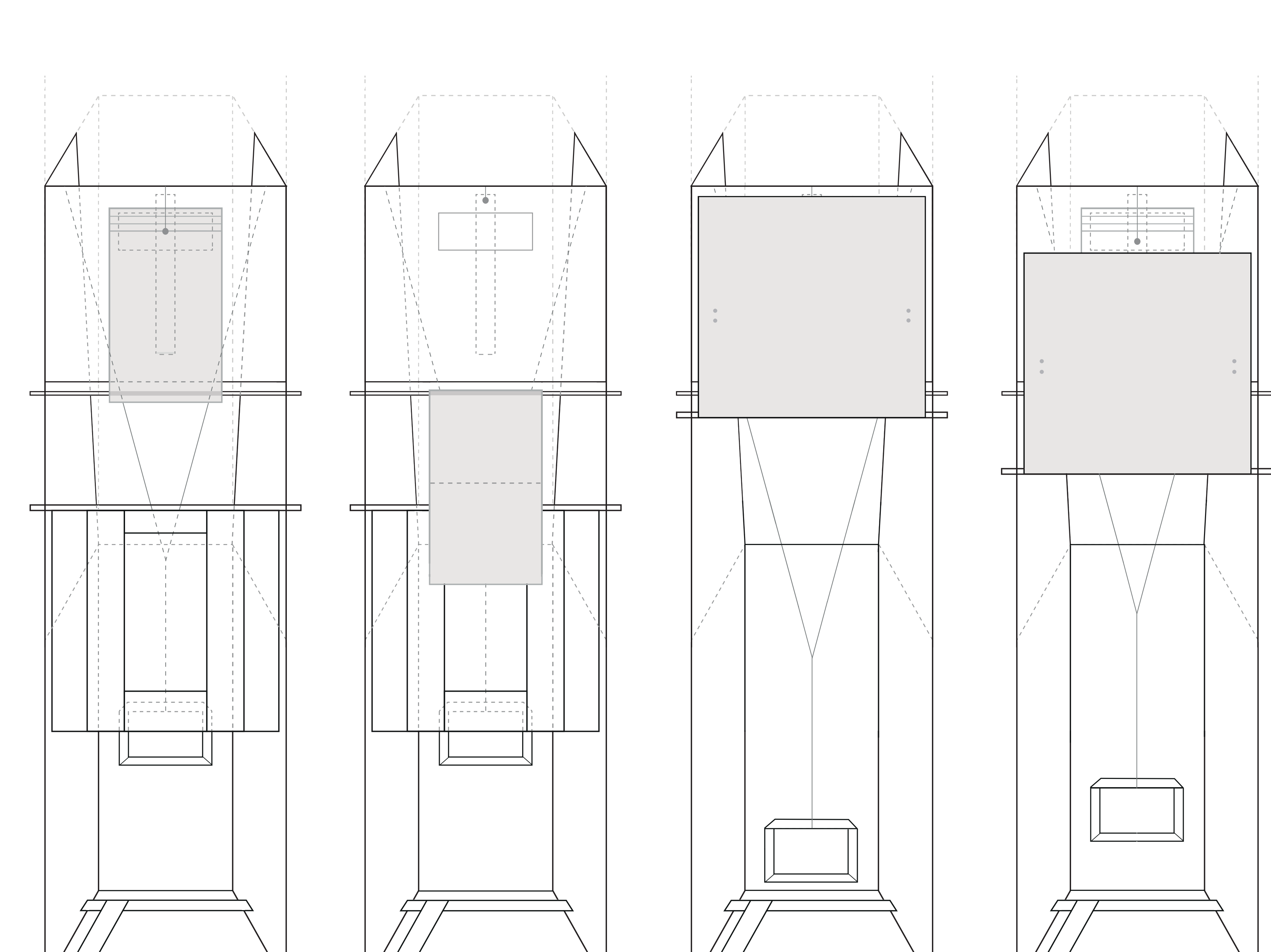
Paso uno: las hojas se encuentran estradas en la zona superior del soporte, presionadas entre el imán y la cinta metálica, esta es la fase donde inicia el hojear.
