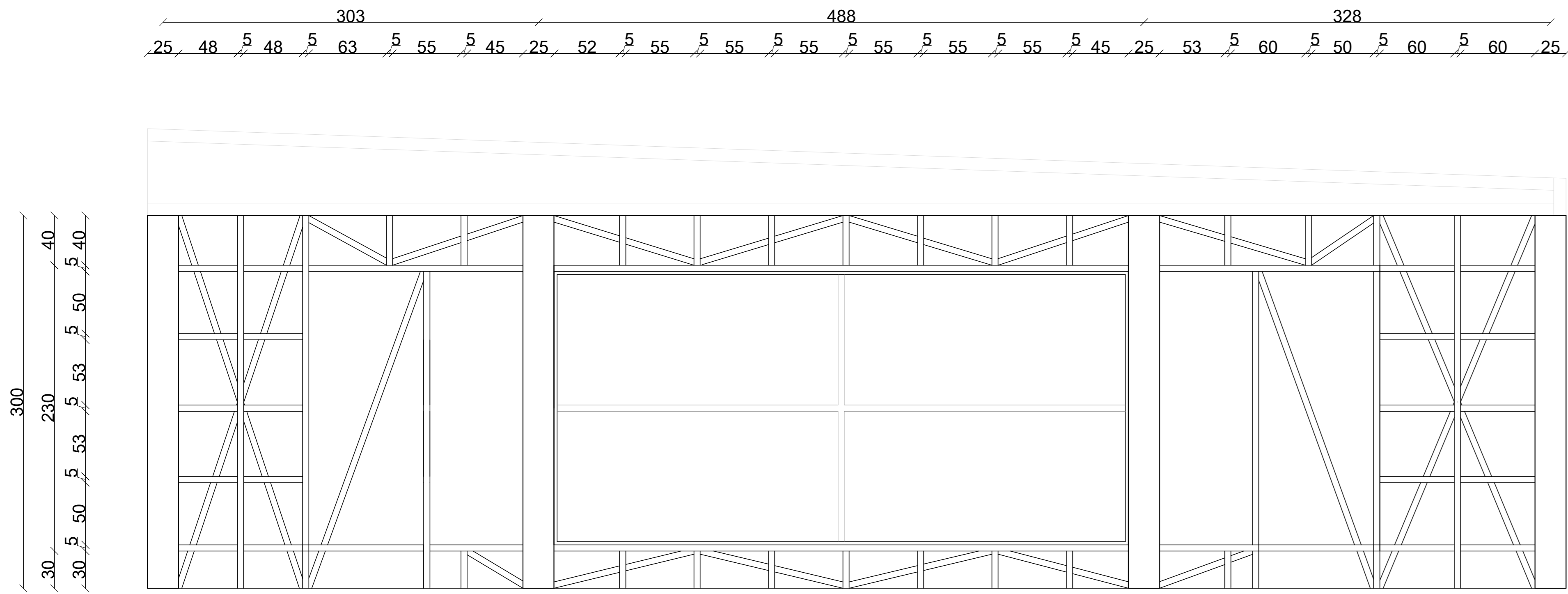
ELEVACION PONIENTE ESCALA. 1/25
