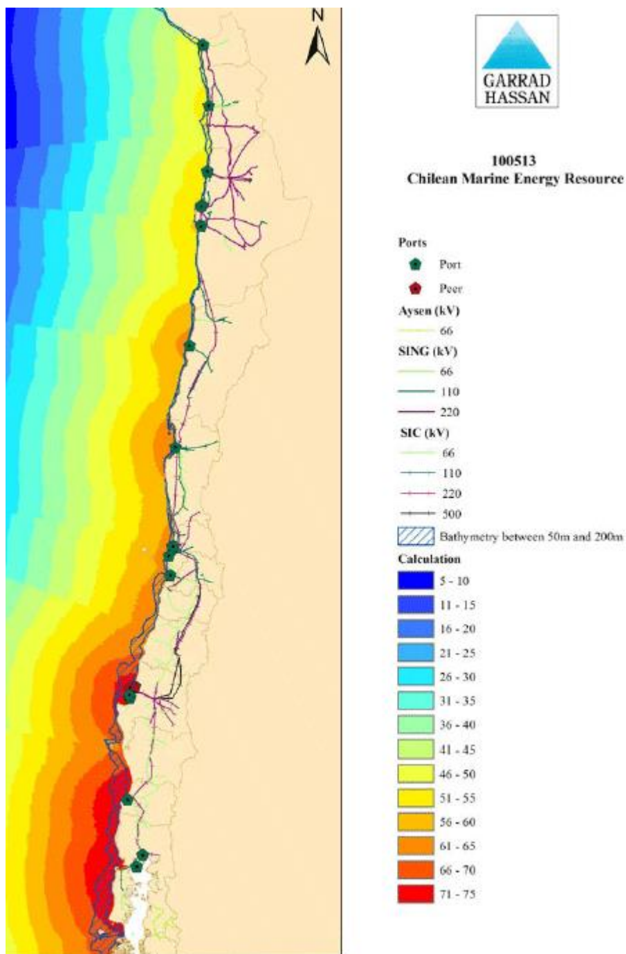
Imagen 3. Potencial de energía undimotriz en Chile.
