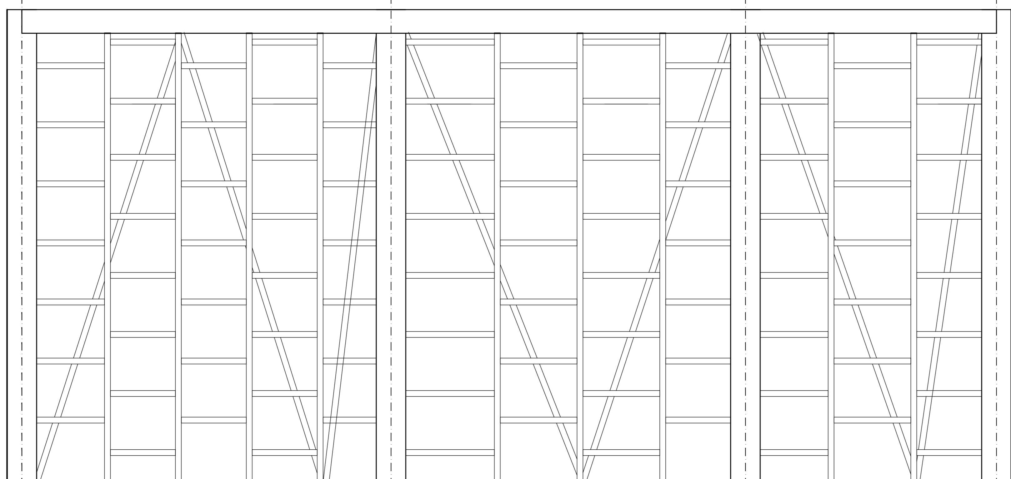
Elevación Este
