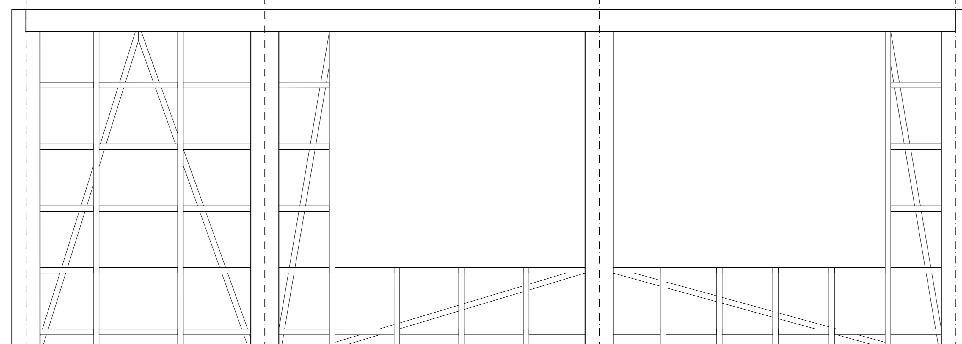
Elevación Oeste
