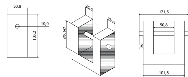
(3) Pieza C viga
