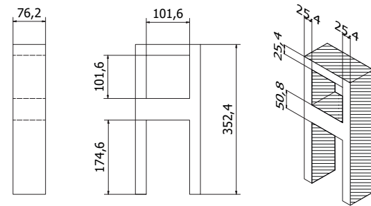
(4) Pieza C
