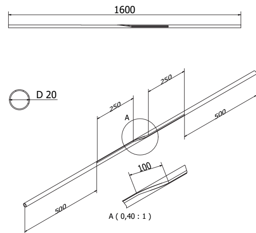
(2) Tubo 2
