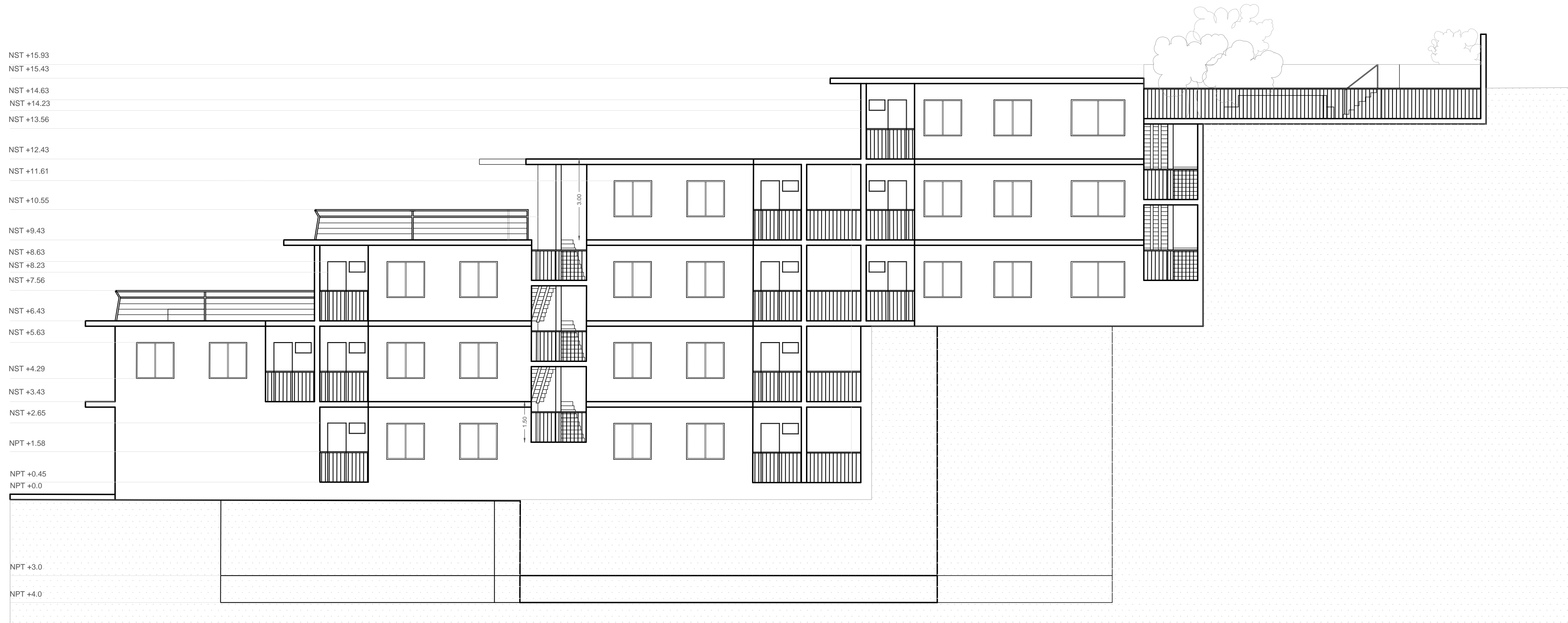
ELEVACIÓN PONIENTE ESCALA 1:100
