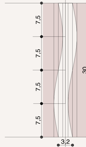
Figura 5 Dimensionamiento Andamios Planimetría 1:5
