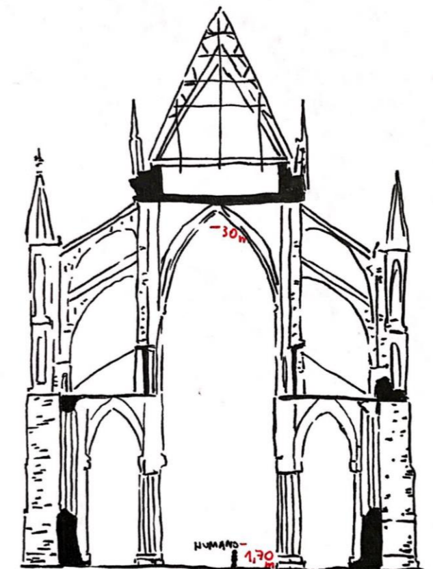
SECCIÓN TRANSVERSAL
