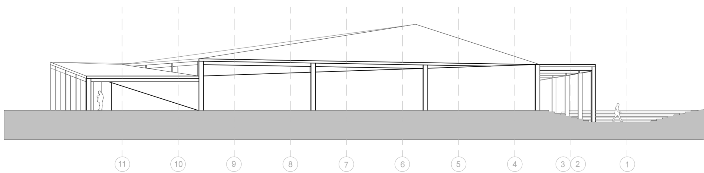
ELEVACIÓN ESTE
