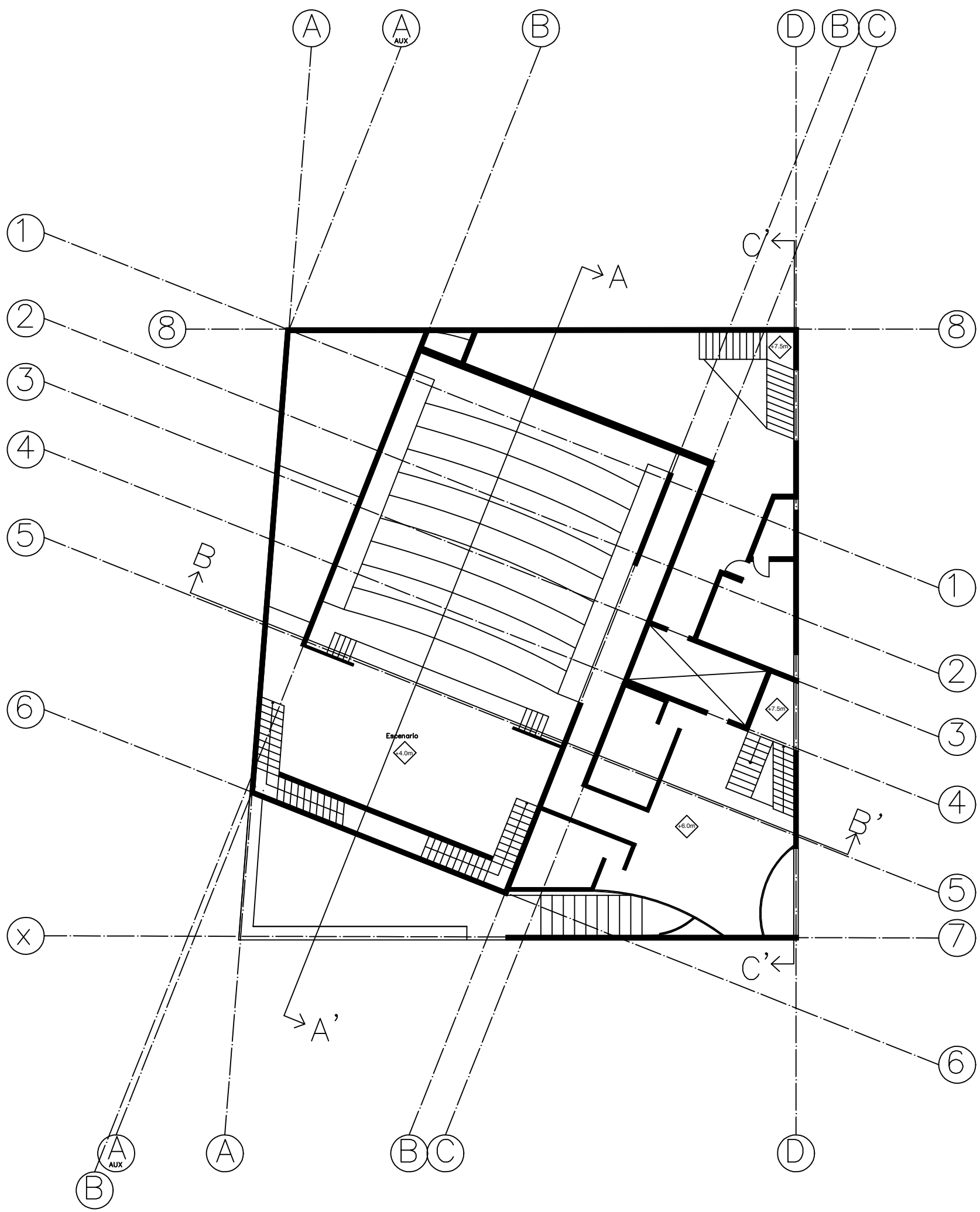
Planta 2
