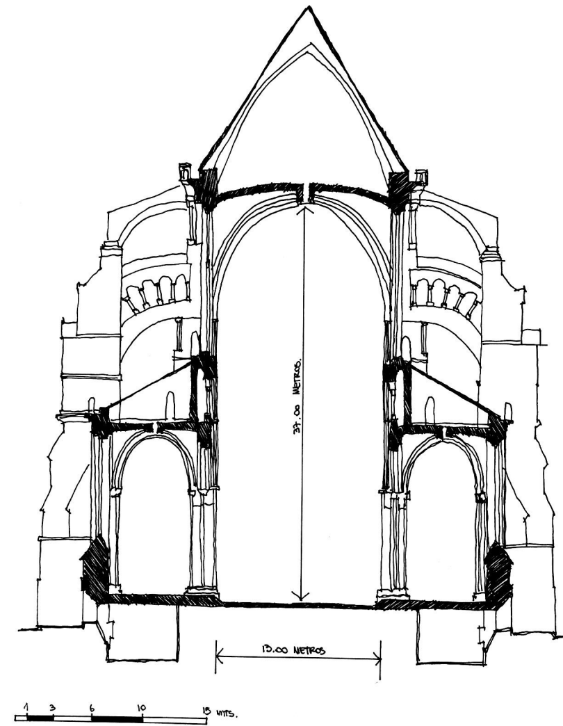
2/ Corte Transversal
