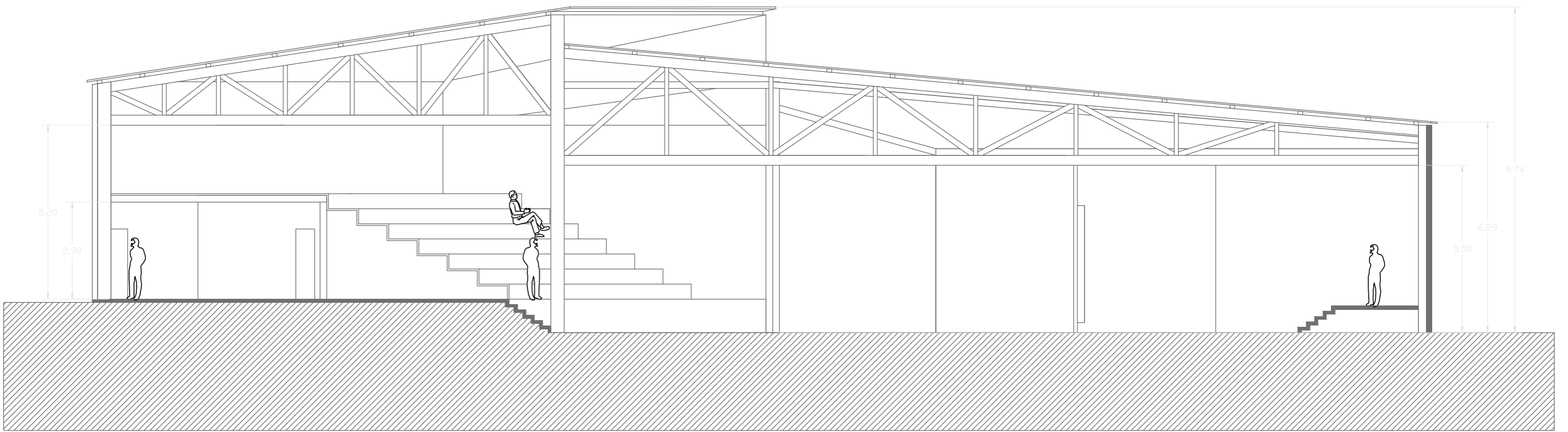
Corte B-B'
