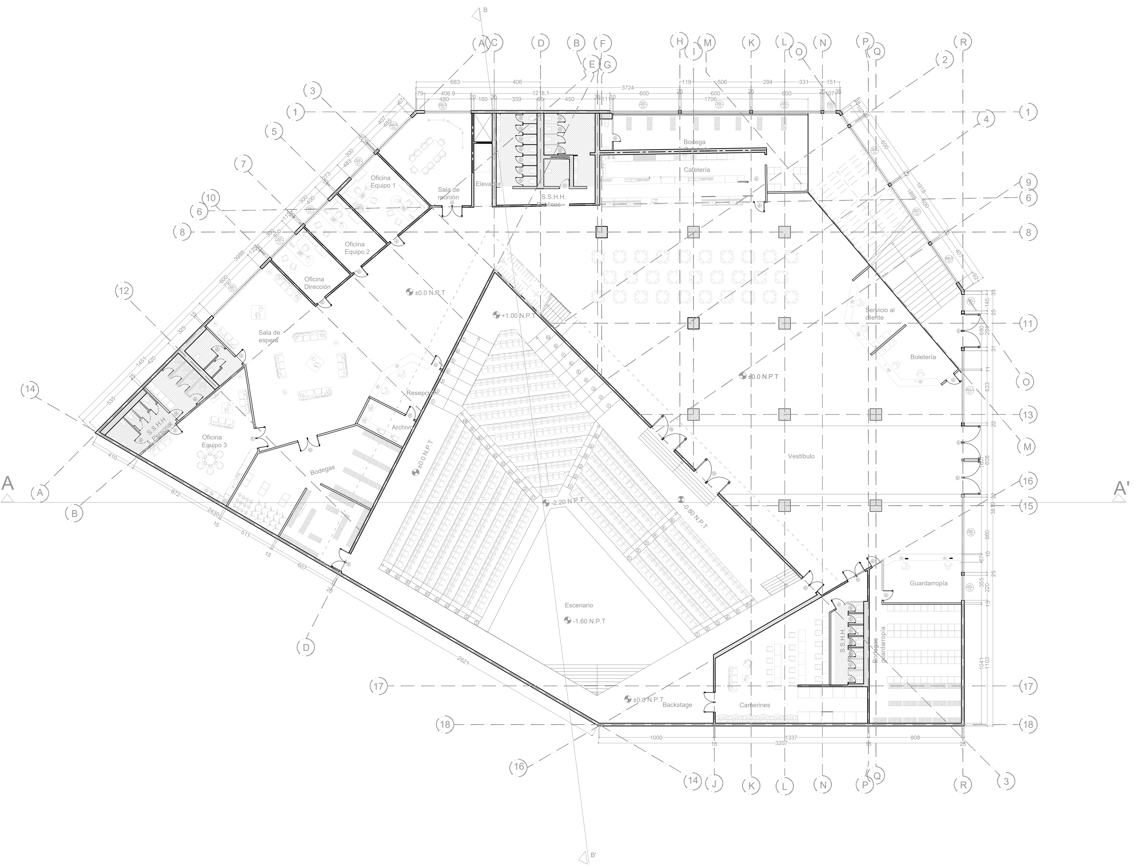
PLANO ARQUITECTURA NIVEL 1 ESC 1:200
