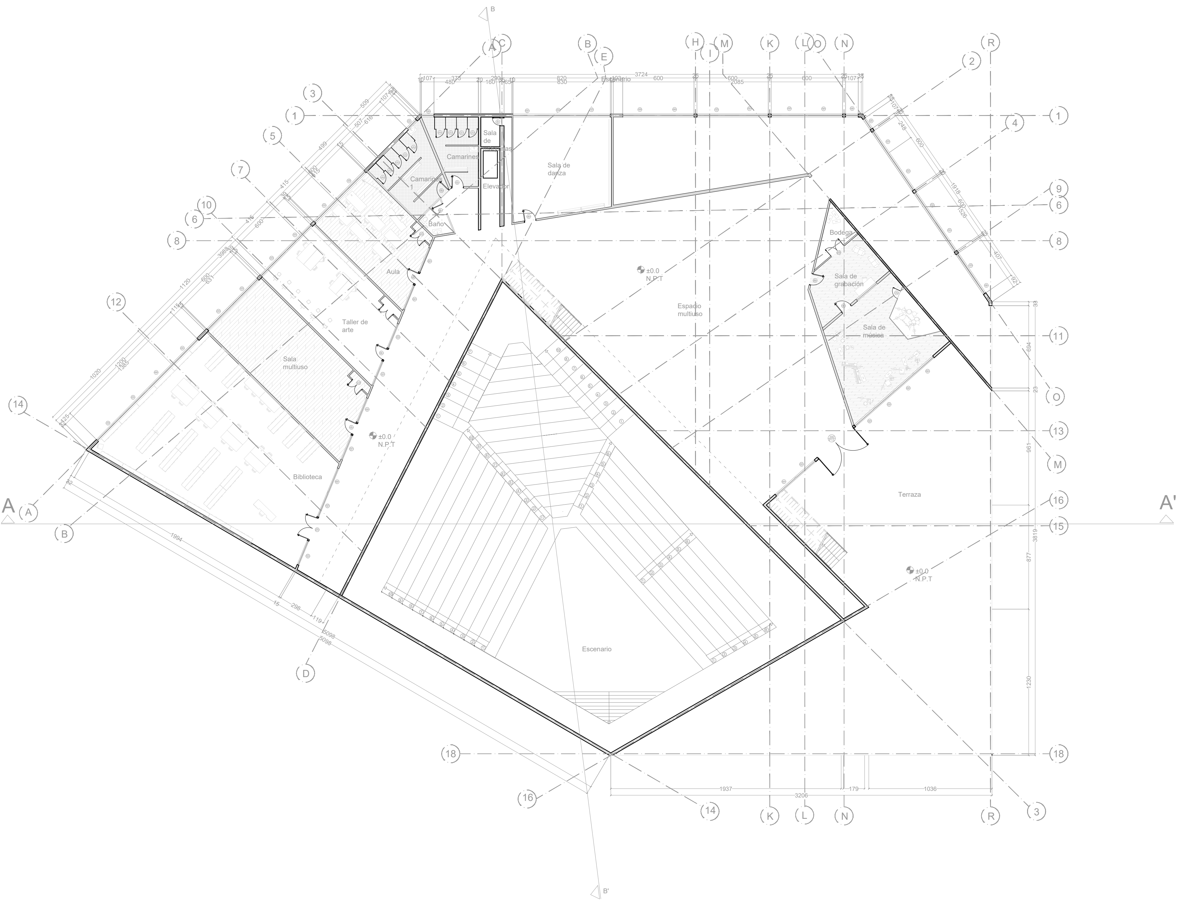
PLANO ARQUITECTURA NIVEL 2 ESC 1:200
